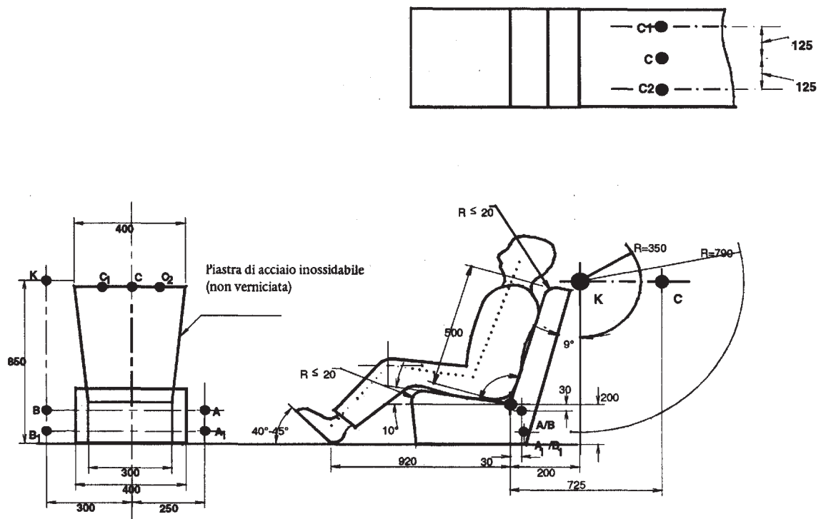
Figura 1 CARRELLO, SEDILE, ANCORAGGIO
