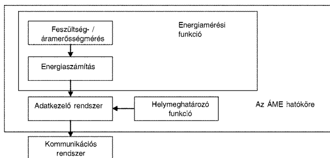
Az villamos fogyasztásmérő készülék funkcionális ábrája
