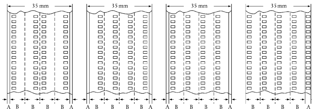
Példák több képsávú filmekre
