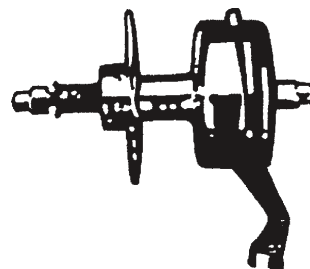
Kontra dobfék
