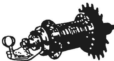
Lábbal működtetett kontrafék
