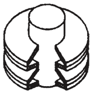
Korongos rugórendszer (metszet)
