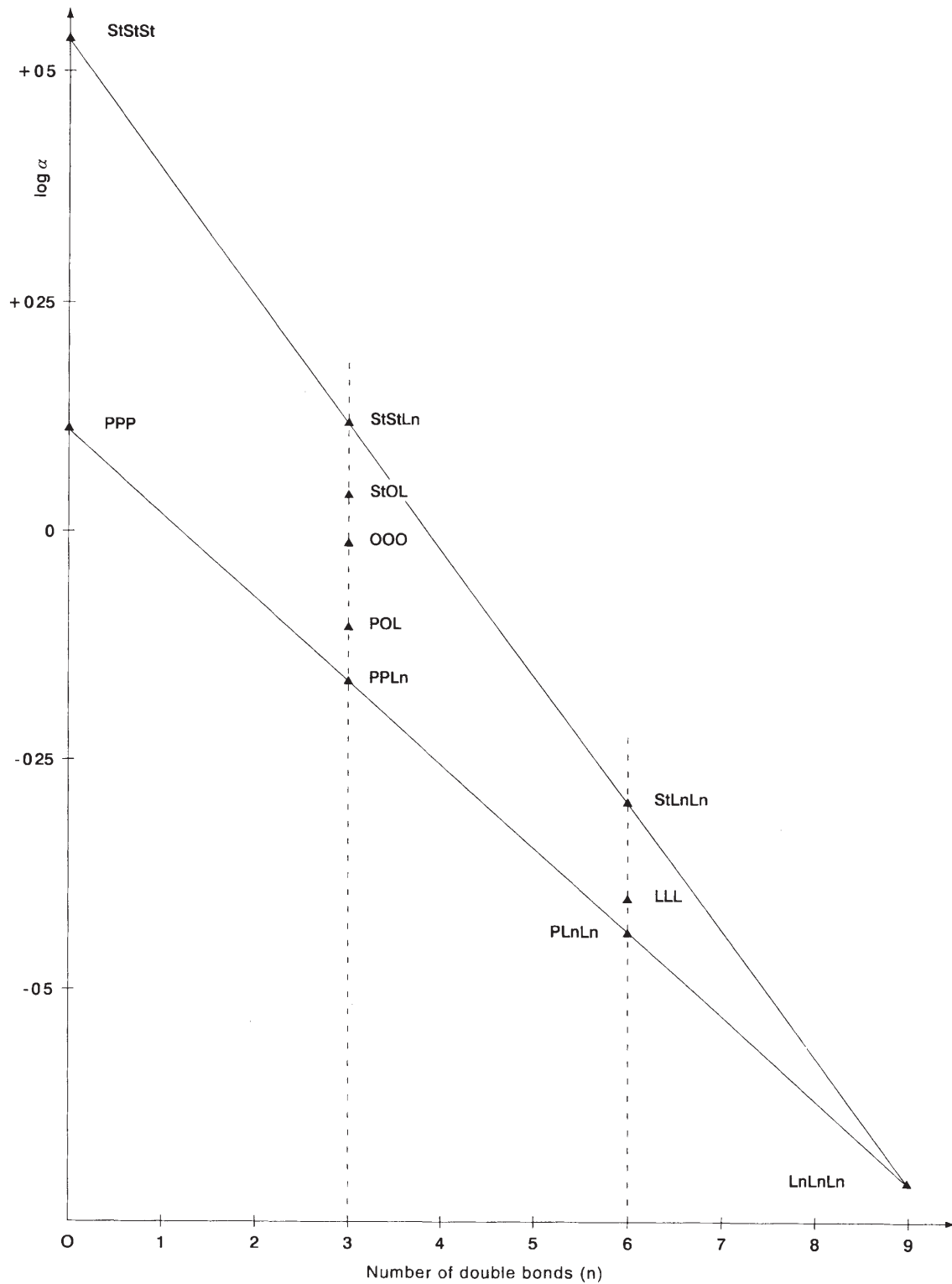
1. ábra: A \log \alpha és f (kettős kötések száma) grafikonja
