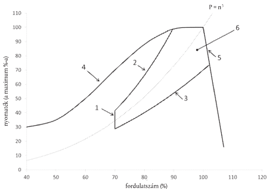
Az E3. NRSC-ciklussal vizsgált motorok ellenőrzési tartománya
