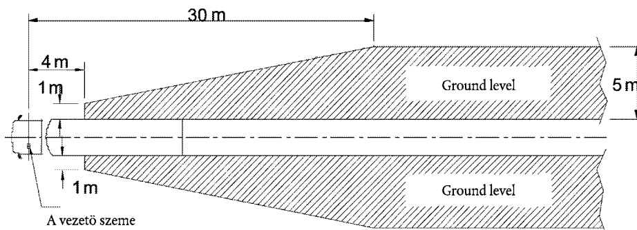
7. ábra: A II. osztályba tartozó tükör látótere
