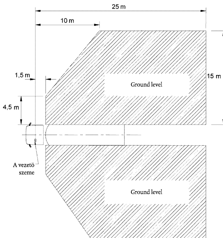
9. ábra: A IV. osztályba tartozó széles látószögű tükrök látótere
