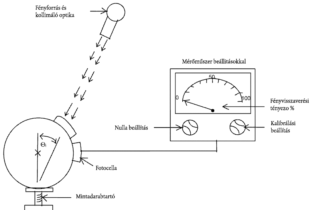
4. ábra: Általános reflektométer a két kalibrálási módszerre mutatja be a kísérlet felállítását
