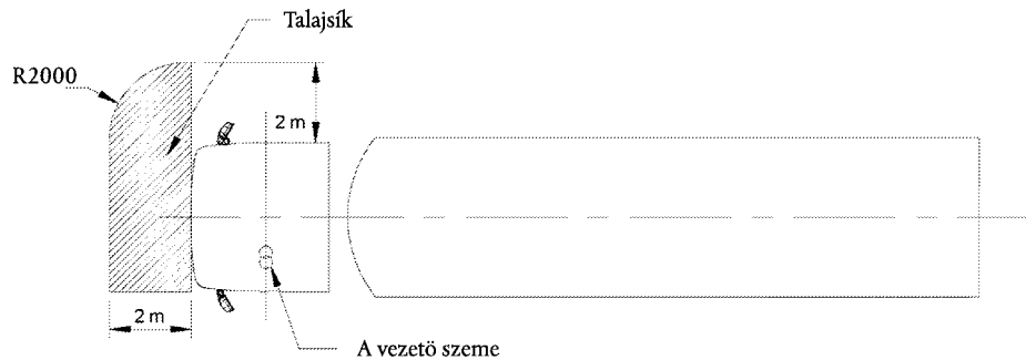
11. ábra: A VI. osztályba tartozó mellső tükör látótere
