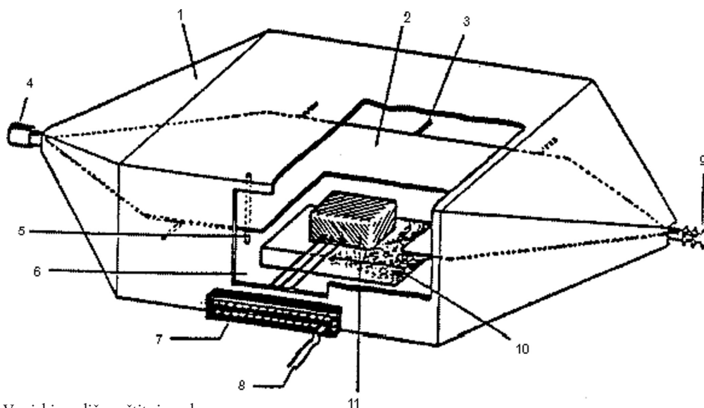
Ispitivanje TEM kavezom
