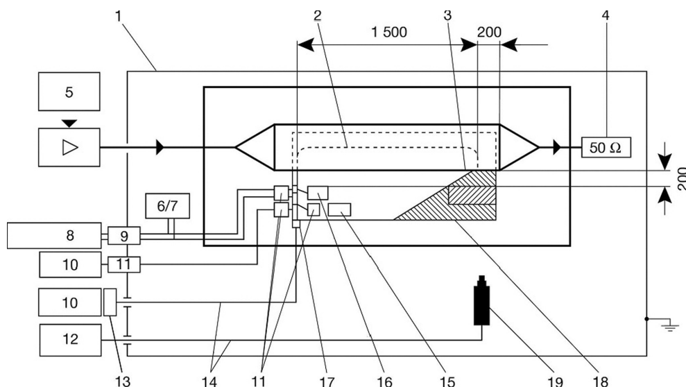
Ispitivanje trakastim vodom od 150 mm
