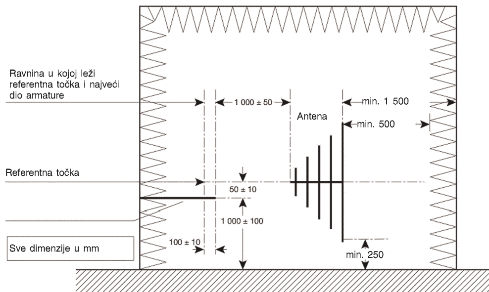
Pogled s ispitnog stola u ravnini uzdužne simetrije
