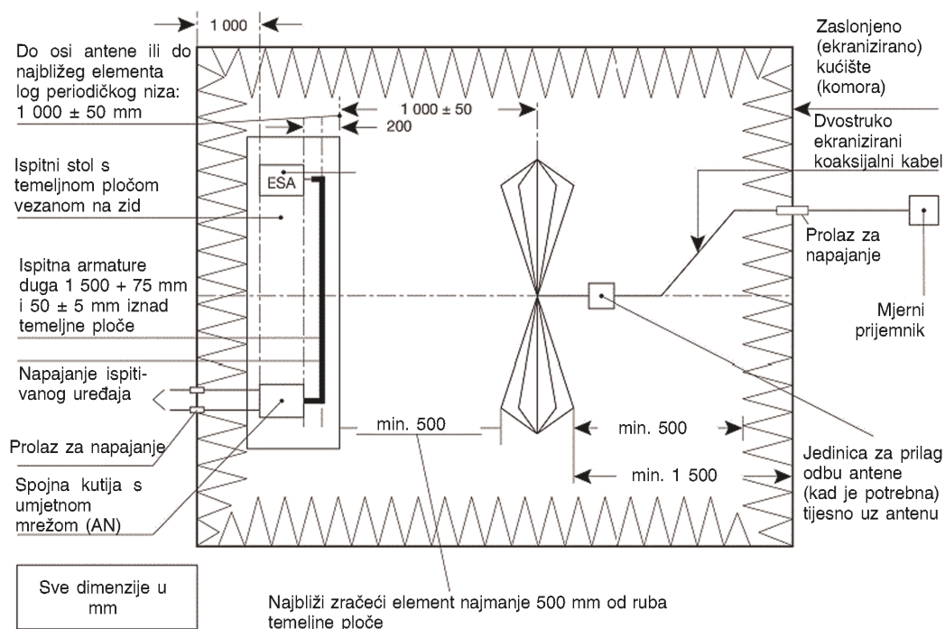
Ispitni raspored (opći izgled)
