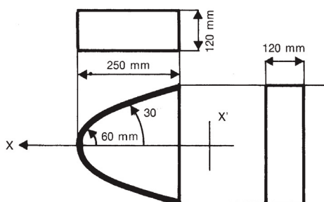
Crtež naprave
