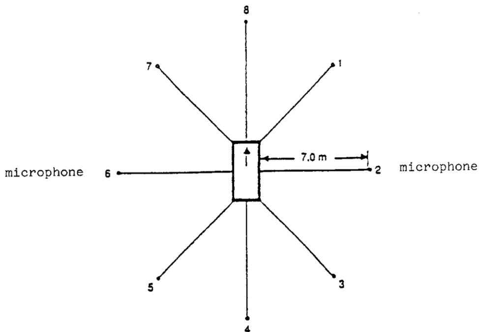
Slika 1.: Položaji mikrofona pri mjerenju buke komprimiranog zraka
