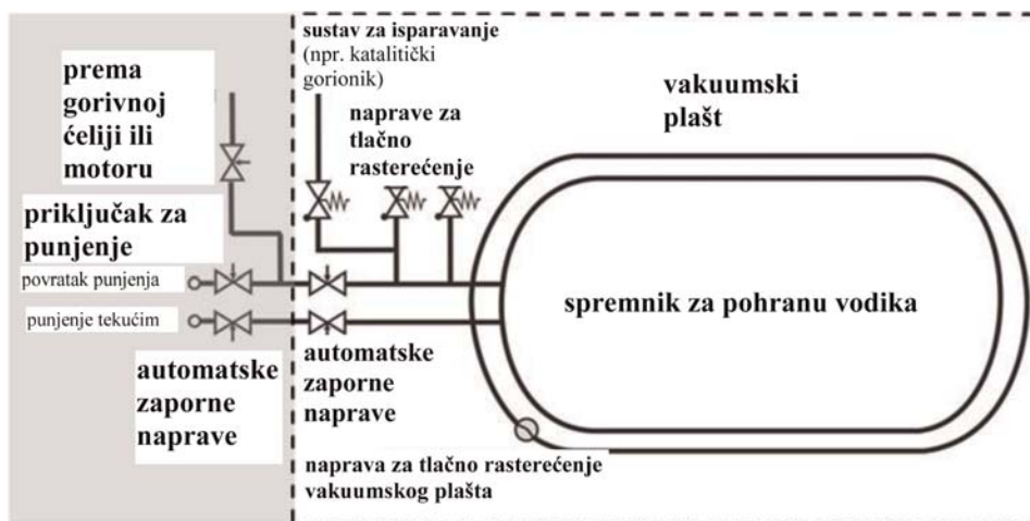
Tipičan sustav za pohranu ukapljenog vodika
