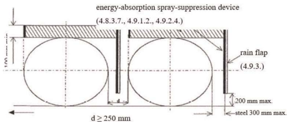
(b) Pojedinačne osovine s razmakom između guma koji nije manji od 250 mm
