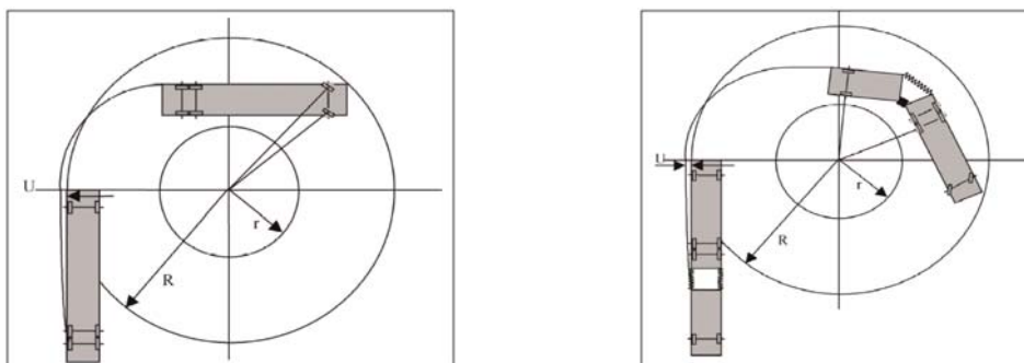
Slika 2.a.: zaokret prema stražnjem dijelu (vozila osim zglobnih autobusa)
