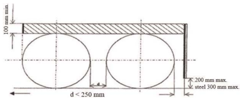
(a) Višestruke osovine s razmakom između guma manjim od 250 mm
