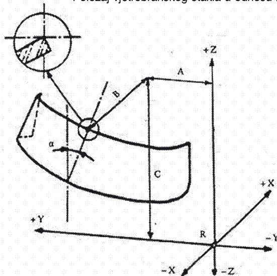
Položaj vjetrobranskog stakla u odnosu na indeksnu točku
