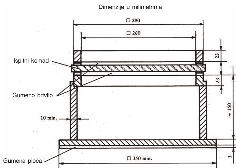
Slika 1. — Stalak za ispitivanja kuglom
