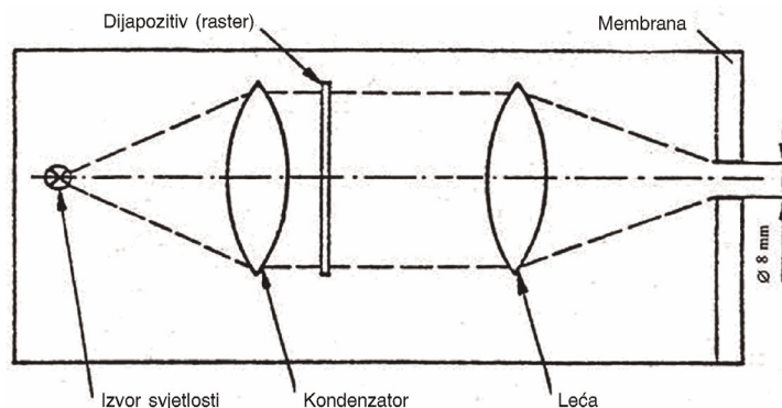
Slika 7. — Optički razmještaj projektora
