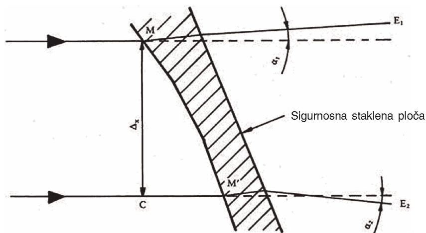
Slika 6. — Dijagramski prikaz optičkog iskrivljenja
