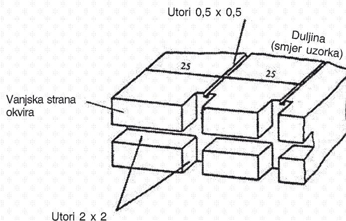
Slika 19. — Primjer presjeka donje konstrukcije okvira u obliku slova U za žičanu potpornu instalaciju
