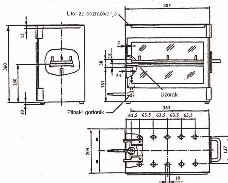
Slika 16. — Primjer komore za izgaranje
