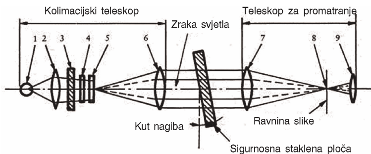
Slika 12. — Razmještaj pribora
