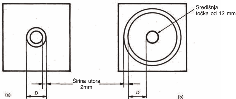
Slika 11. — Dimenzije meta
