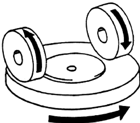
Slika 4. — Dijagram instrumenta za brušenje
