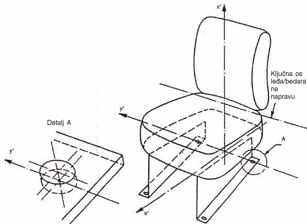
Slika 11. Utvrđivanje SIP referentnih osi
