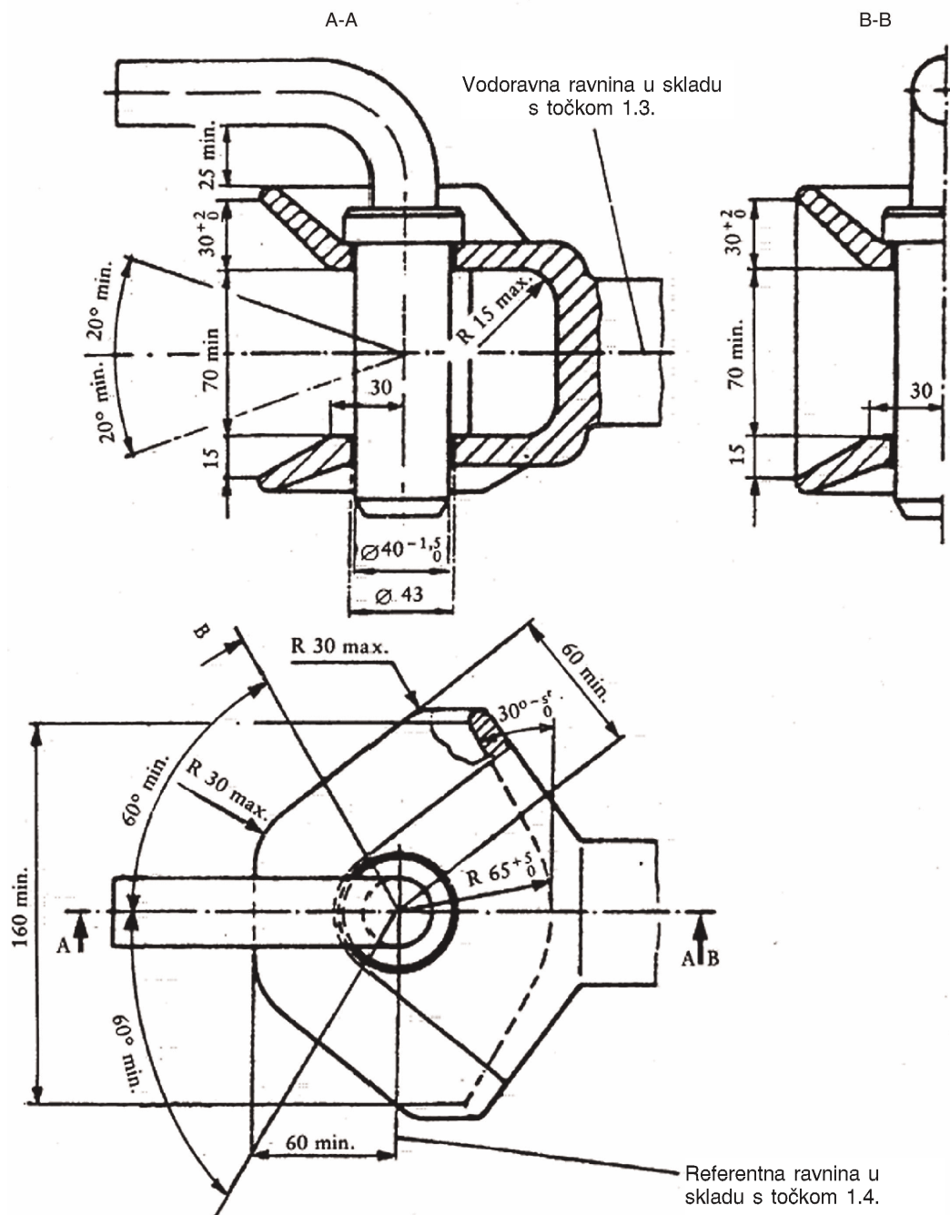
Slika 2. — Neautomatska spojnica za prikolicu
