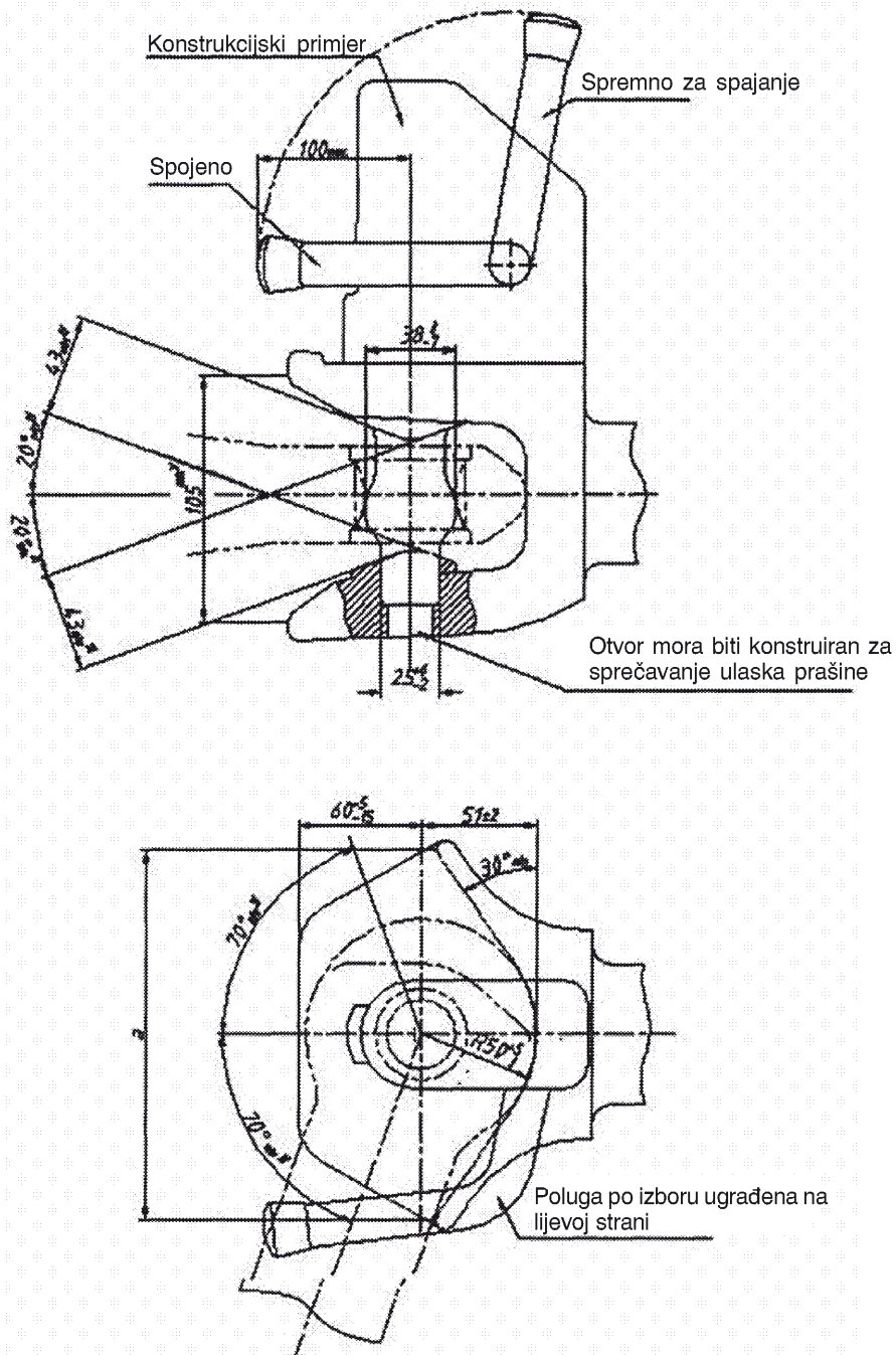
Slika 1.c — Automatska spojnica za prikolicu s izbočenim klinom
