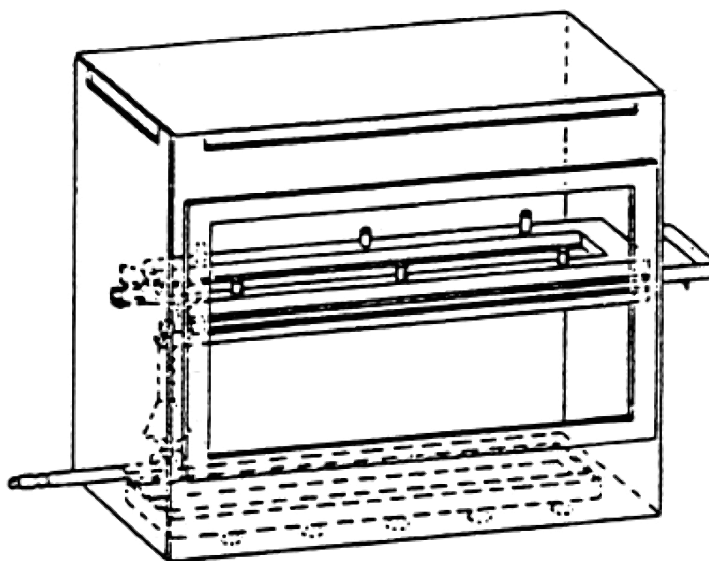
Slika 15. — Primjer komore za izgaranje s držačem uzorka i posudom za kapljevine
