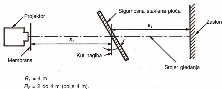
Slika 9. — Razmještaj pribora za ispitivanje optičkog iskrivljenja
