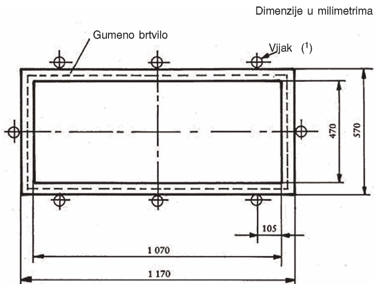
Slika 3. — Stalak za ispitivanje modelom glave
