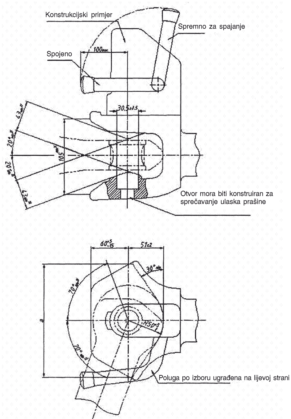
Slika 1.b — Automatska spojnica za prikolicu s cilindričnim klinom
