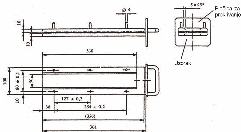
Slika 18. — Primjer držača uzorka
