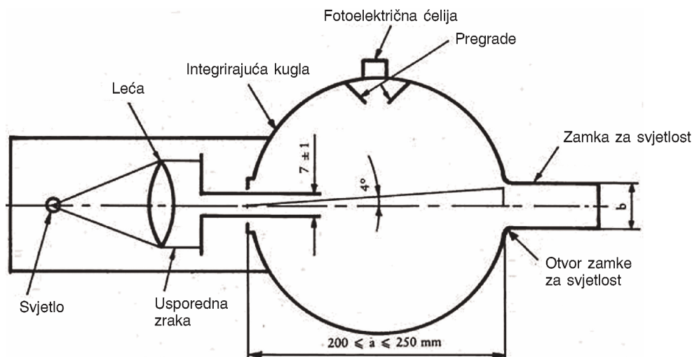
Slika 5. — Hazemetar (mjerac izmaglice)
