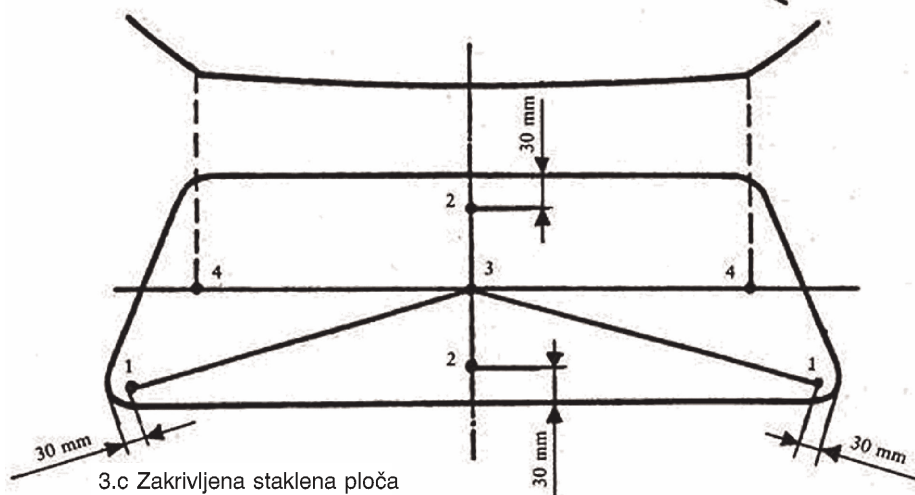
Slike 3.a, 3.b i 3.c — Propisana mjesta udara za jednoliko kaljene staklene ploče
