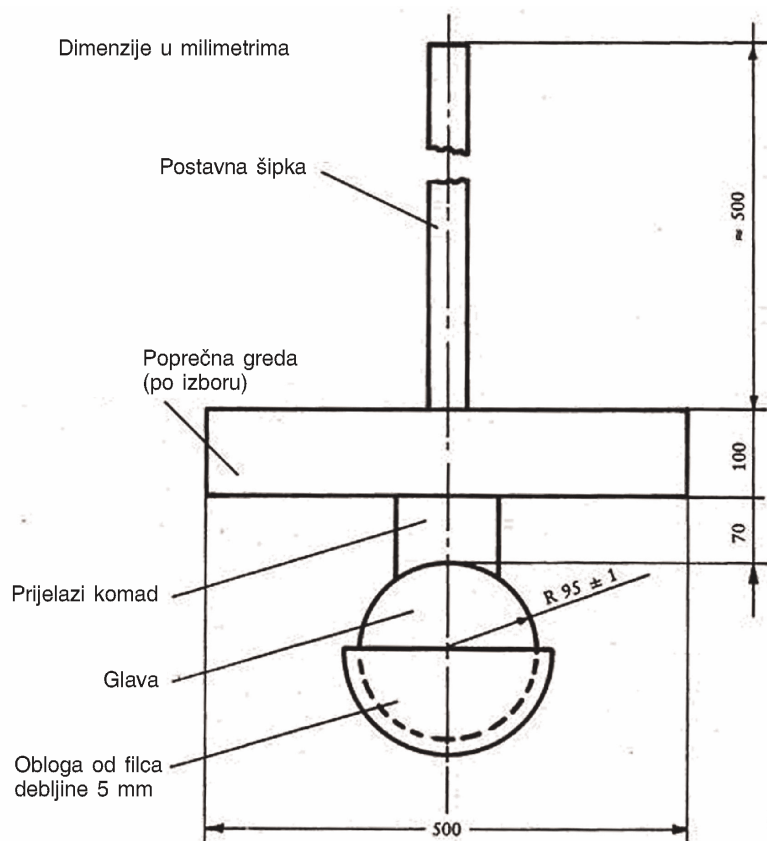
Slika 2. — Težina modela glave
