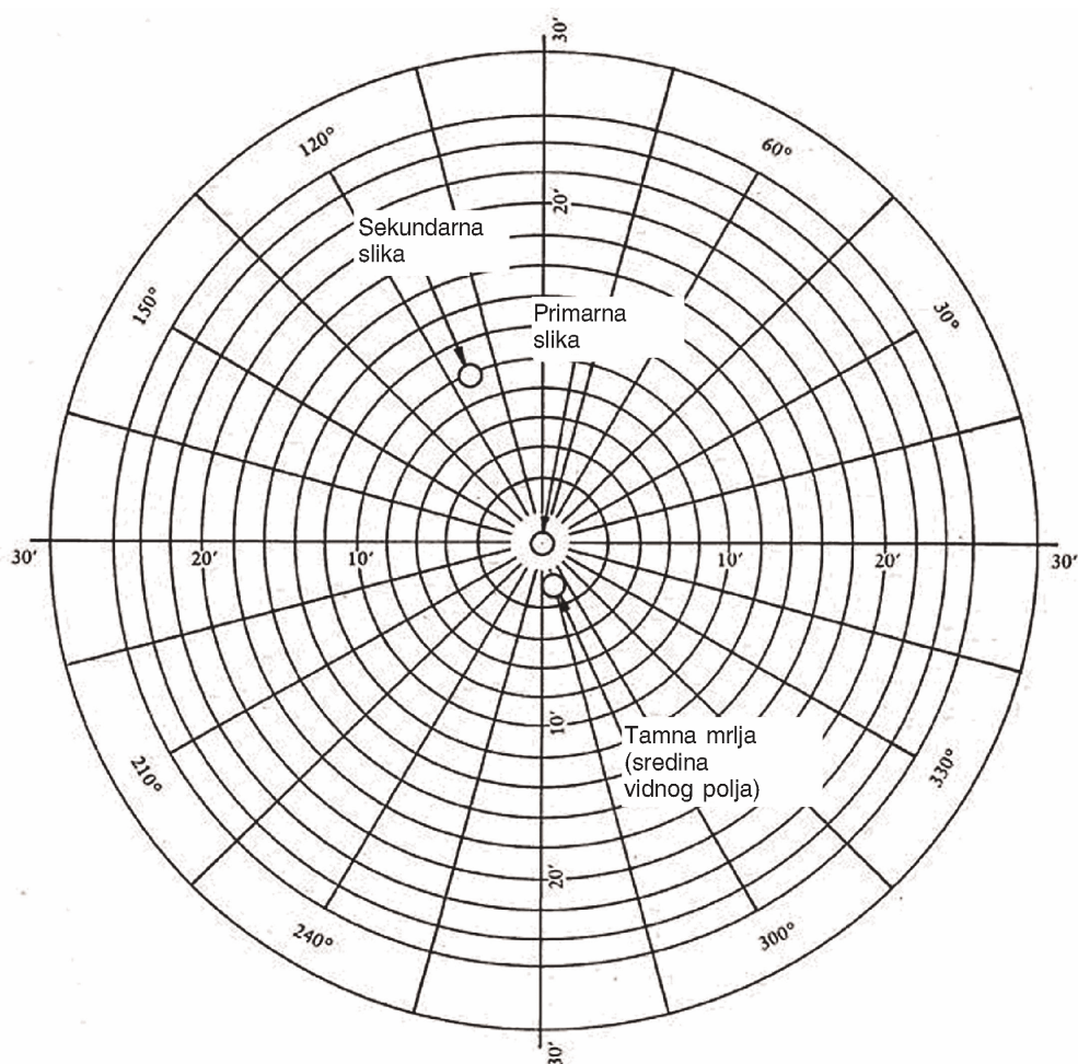
Slika 14. — Primjer promatranja metodom ispitivanja kolimacijskim teleskopom
