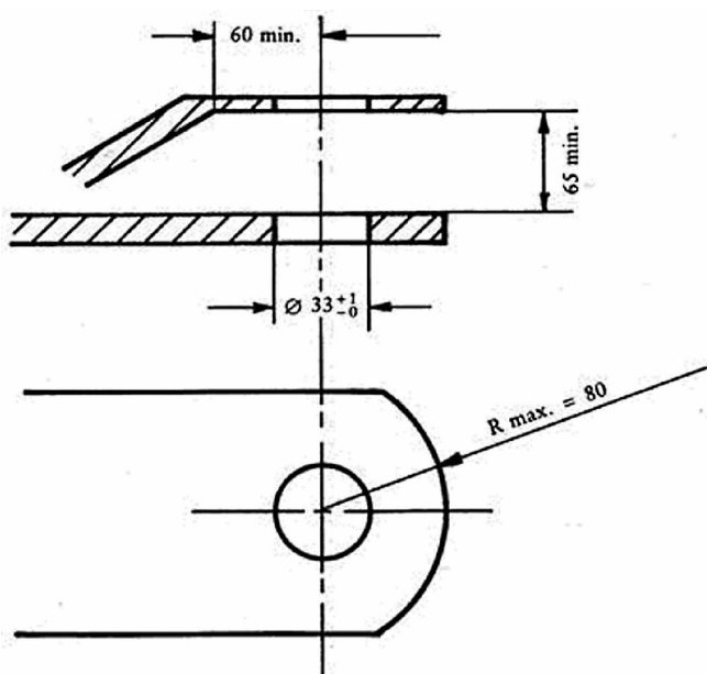
Slika 3. — Traktorska vučna vilica
