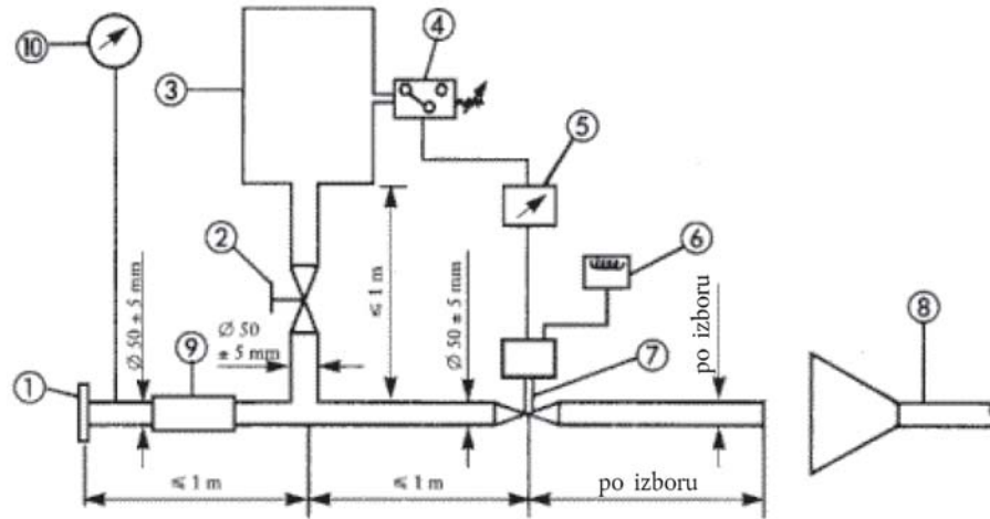
Slika Ap3-4 Ispitni uređaj za kondicioniranje pulziranjem
