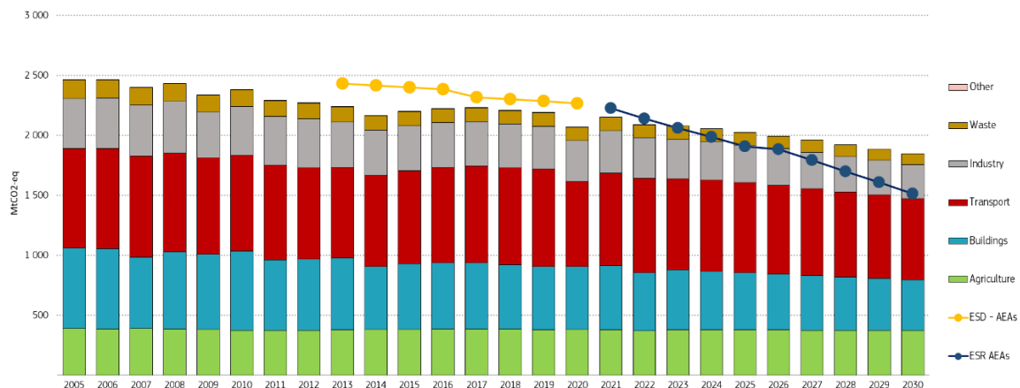
Fíor 10: Astaíochtaí in earnálacha a chumhdaítear le reachtaíocht comhroinnte díchill 2005-2030 agus leithdháiltí bliantúla astaíochtaí, AE-27 60
