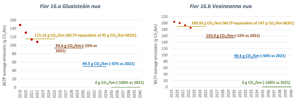
Fíor 16: Meánastaíochtaí CO 2 (poncanna) agus spriocanna (línte) le haghaidh fhlít uile an Aontais i gcás gluaisteáin nua (ar chlé) agus veaineanna nua (ar dheis).
