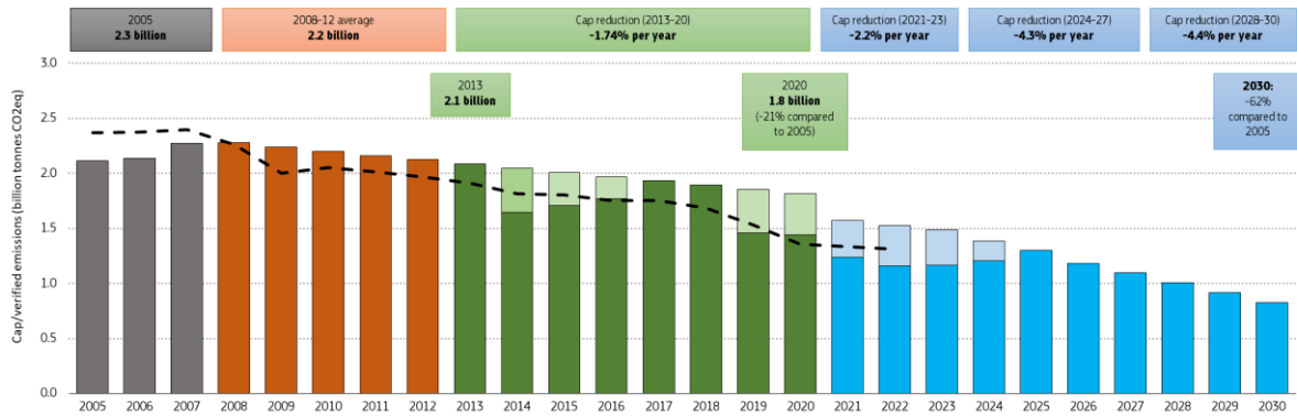
Fíor8: Astaíochtaí CTA fíoraithe 2005-2022, réamh-mheastacháin na mBallstát le bearta 2021-2030, céimeanna caidhpe CTA 2, 3 agus 4, agus barrachas carntha de lamháltais CTA 2008-2021 lena n-áirítear an Ríocht Aontaithe (Tuaisceart Éireann), an Iorua agus an Íoslainn NB: coigeartaigh i leith chéim chaidhpe 4 54 .
