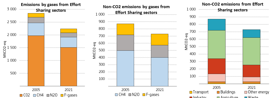
Fíor 13: Astaíochtaí neamh-CO 2 faoi ESR in 2005 agus 2021, de réir earnála agus de réir an chineáil gáis.
