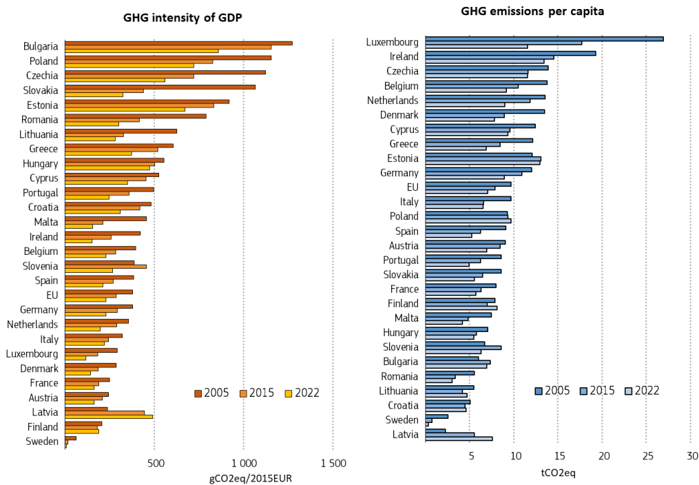
Fíor 5: Déine GCT OTI agus astaíochtaí GCT per capita de réir na mBallstát
