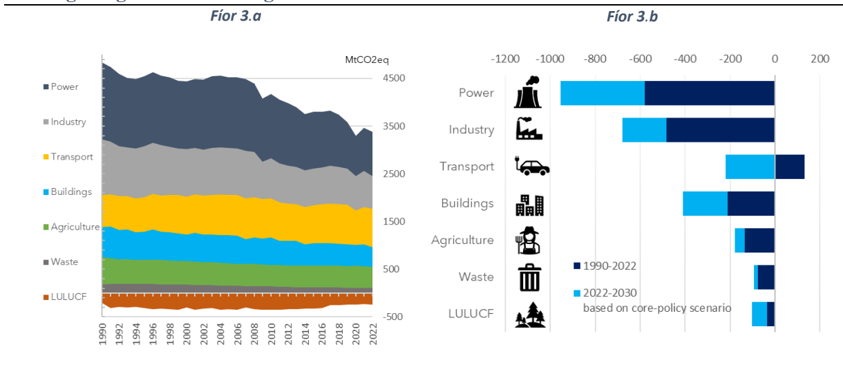
Fíor 3: Astaíochtaí agus aistrihe GCT an Aontais de réir earnála, treochtaí san am a chuaigh thart agus laghduithe a cheanglaítear 23
