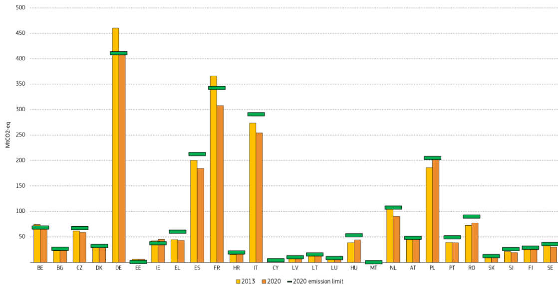
Fíor 11: Athrú ar astaíochtaí ESD idir 2013 agus 2020, in aghaidh leithdháiltí bliantúla astaíochtaí 2020 63
