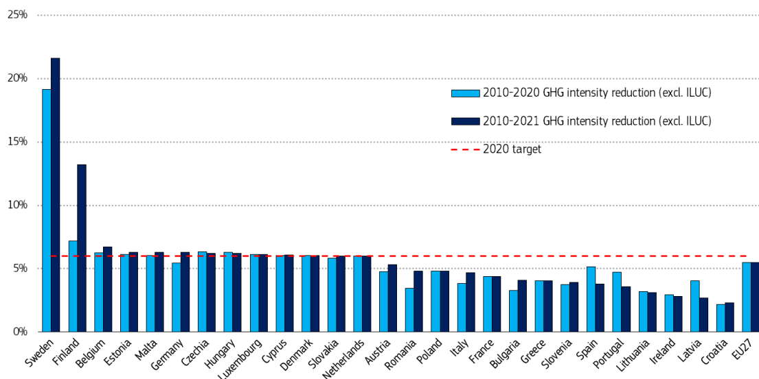
Fíor 17: Lagduithe ar dhéine astaíochtaí GCT breoslaí a bhain soláthróirí breosla an Aontais amach in AE-27, 2010-2020 agus 2010-2021 (Foinse: EEA)
