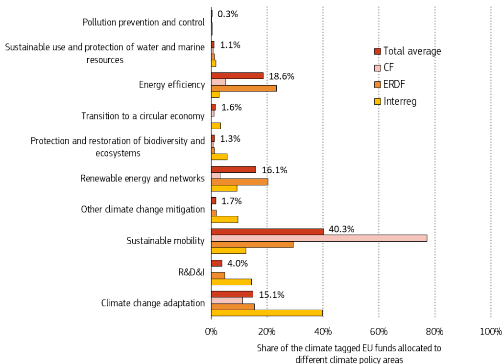
Fíor 24: Méideanna cistí CFRE, CC agus an chomhair chríochaigh Eorpaigh a chaitheann an tAontas ar an aeráid de réir réimse beartais 137
