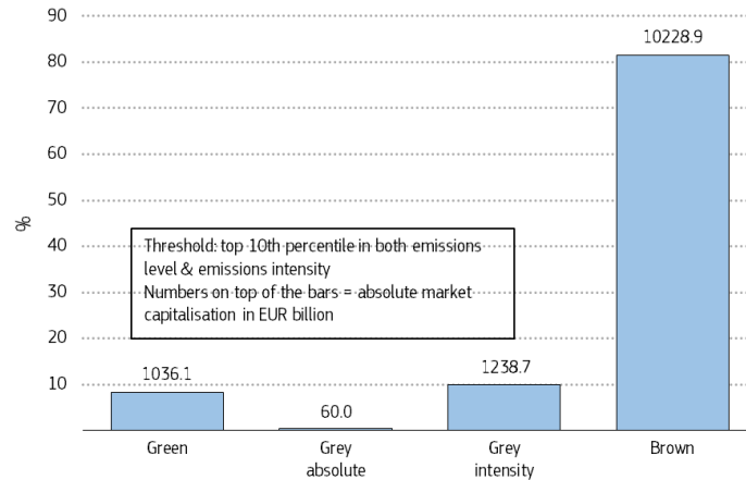
Fíor 23: Caipitliú mhargadh an Aontais de réir glaise, 2021 129
