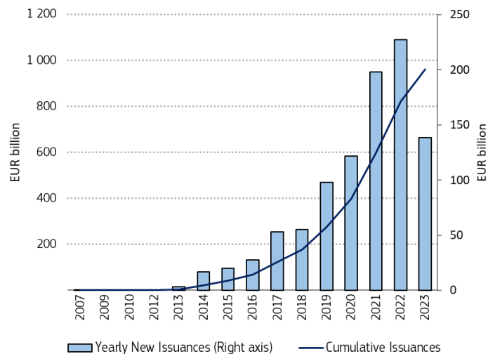
Fíor 19: Eisiúint Bannaí Glasa san Aontas arna n-ailíniú le prionsabail ICMA um bannaí glasa (méideanna) 121
