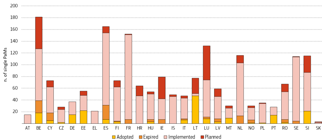
Fíor 14: An líon beartas agus beart aonair a thuairiscigh na Ballstáit i gcás earnáil ESR 76
