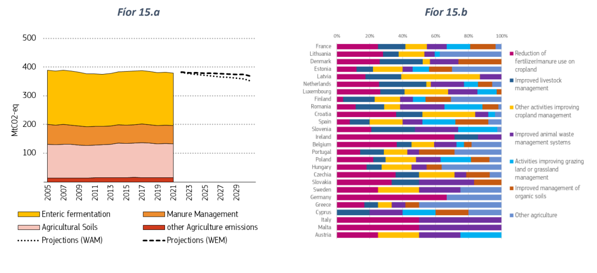
Fíor 15: Astaíochtaí GCT in earnáil na talmhaíochta (AE, 2005-2021) agus beartais agus bearta 2023 arna dtuairisciú le haghaidh earnáil na talmhaíochta (de réir cuspóirí)
