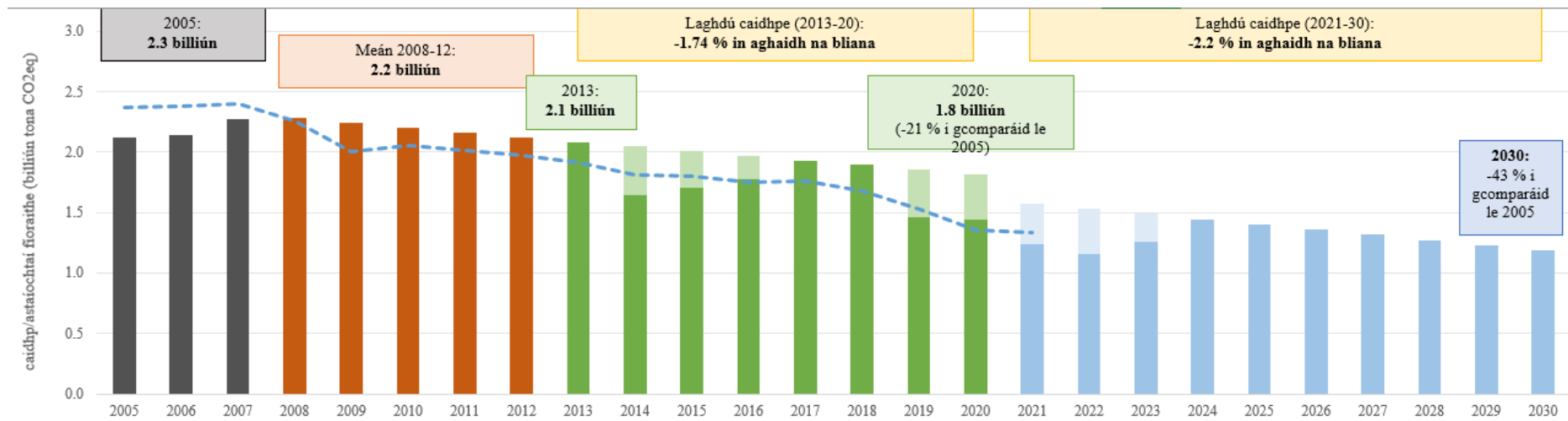
Fíor 1. Caidhp astaíochtaí a shocráítear i CTA an Aontais, i gcomparáid le hastaíochtaí fíoraithe. Eochair eolais: barraí (caidhp), barraí faoi scáth éadrom in 2014-16 (lamháltais arna siarchoinneáil i gcéim 3), barraí faoi scáth éadrom ó 2019 (fothaí lamháltas chuig Cúlchiste Cobhsaíochta an Mhargaidh), líne bhriste (astaíochtaí arna bhfíorú).
