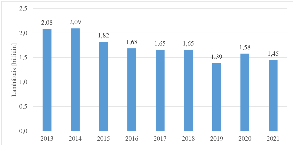
Fíor 5. Barrachas astaíochtaí i CTA an Aontais (2013-21).
