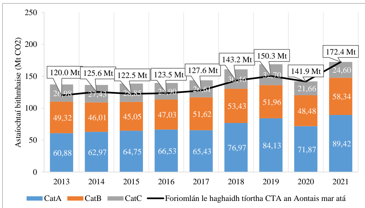
Fíor 4. Astaíochtaí de thionscnamh bithmhais nialas-rátaithe in 2021 i gcomparáid le céim 3 (2013-20). Cuirtear astaíochtaí i láthair ina milliúin tonnaí de choibhéis CO 2 .
