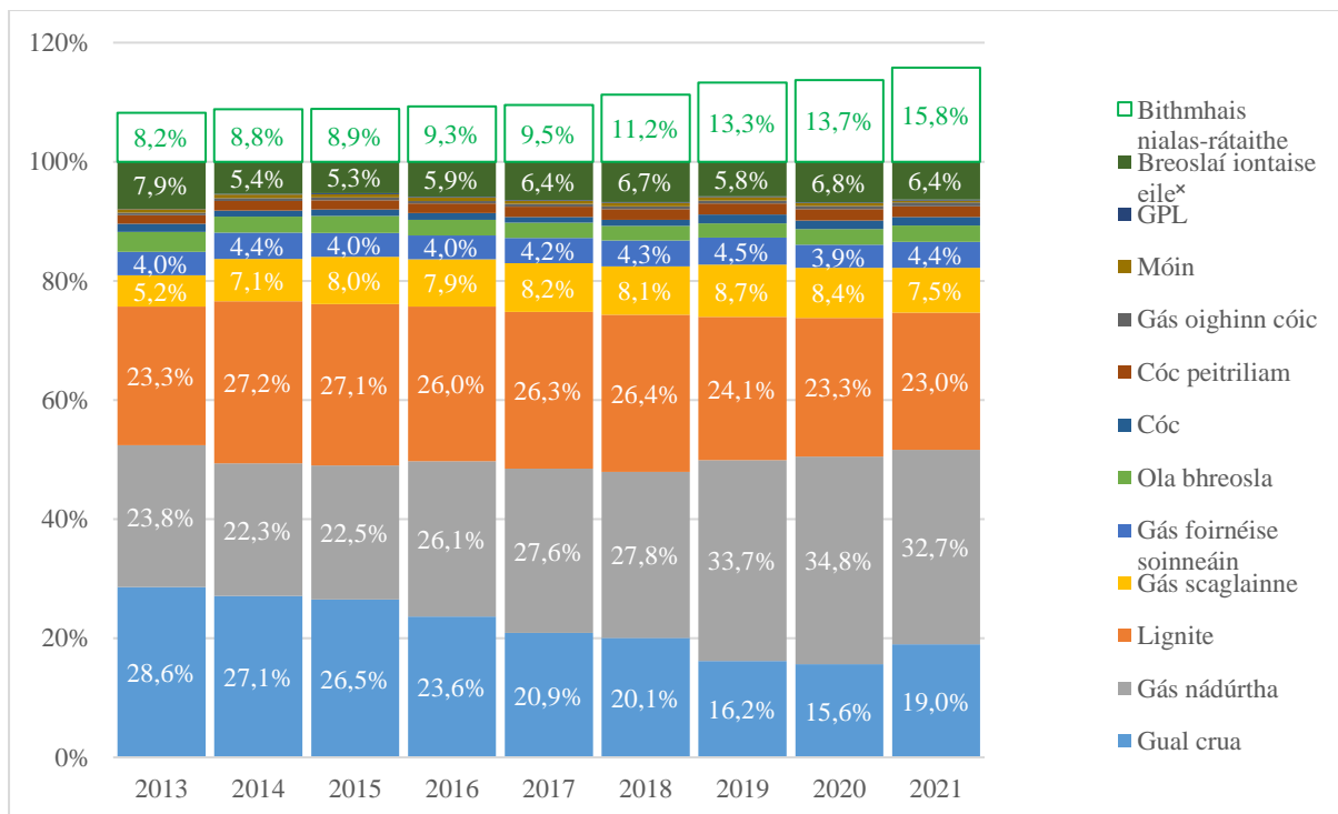
Fíor 3. Astaíochtaí de réir chineál breosla mar sciartha d'astaíochtaí bliantúla breoslaí iontaise. Is ionann agus 100 % na breoslaí iontaise i dteannta a chéile, tagann an bhithmhais sa bhreis air sin. Lipéid nach dtaispeántar mura sáraíonn an breosla 3 % den iomlán, * = nach gcumhdaítear leis na breoslaí sonraithe eile.
