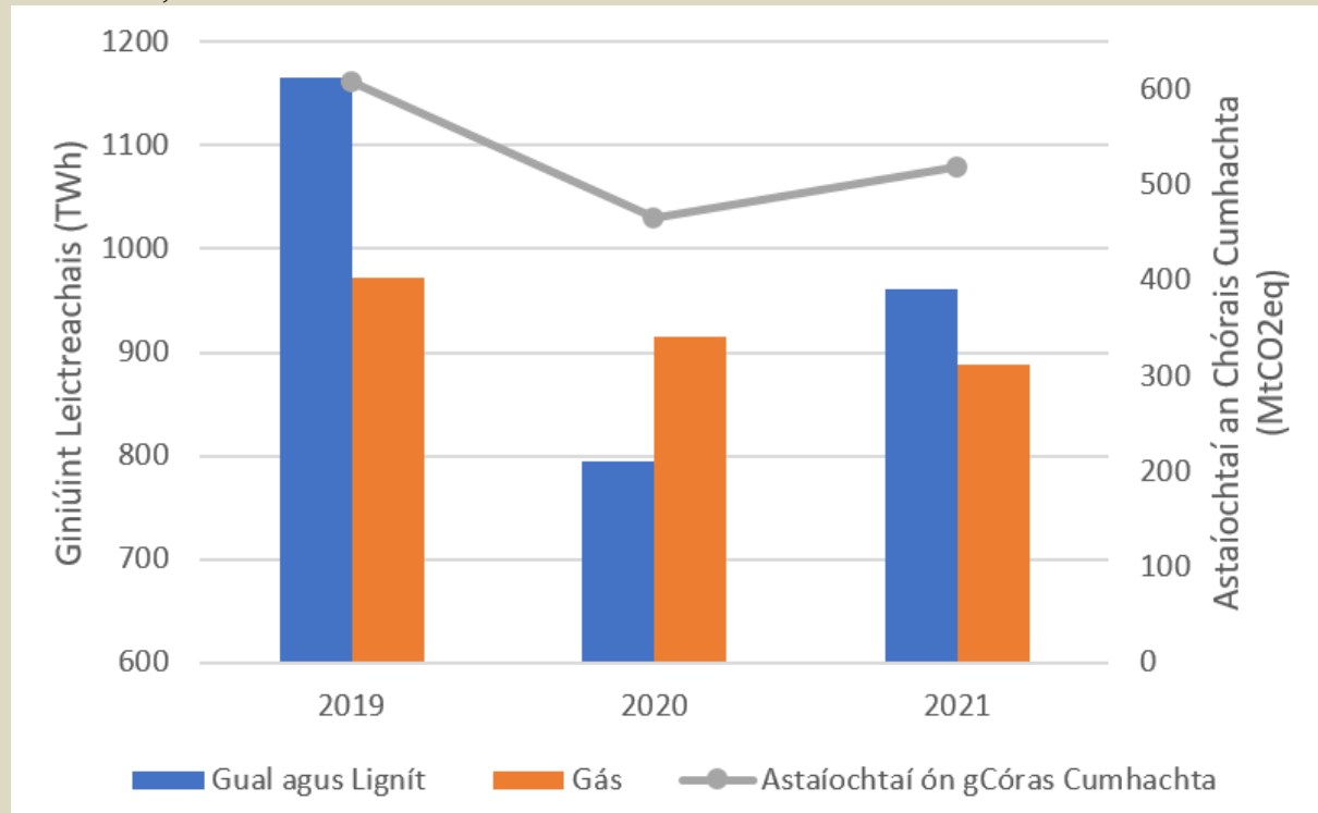
Fíor 3 - Leictreachas arna ghiniúint ag gual, lignít agus gás agus astaíochtaí CO 2 den chóras cumhachta, 2019-2021 (d) .
