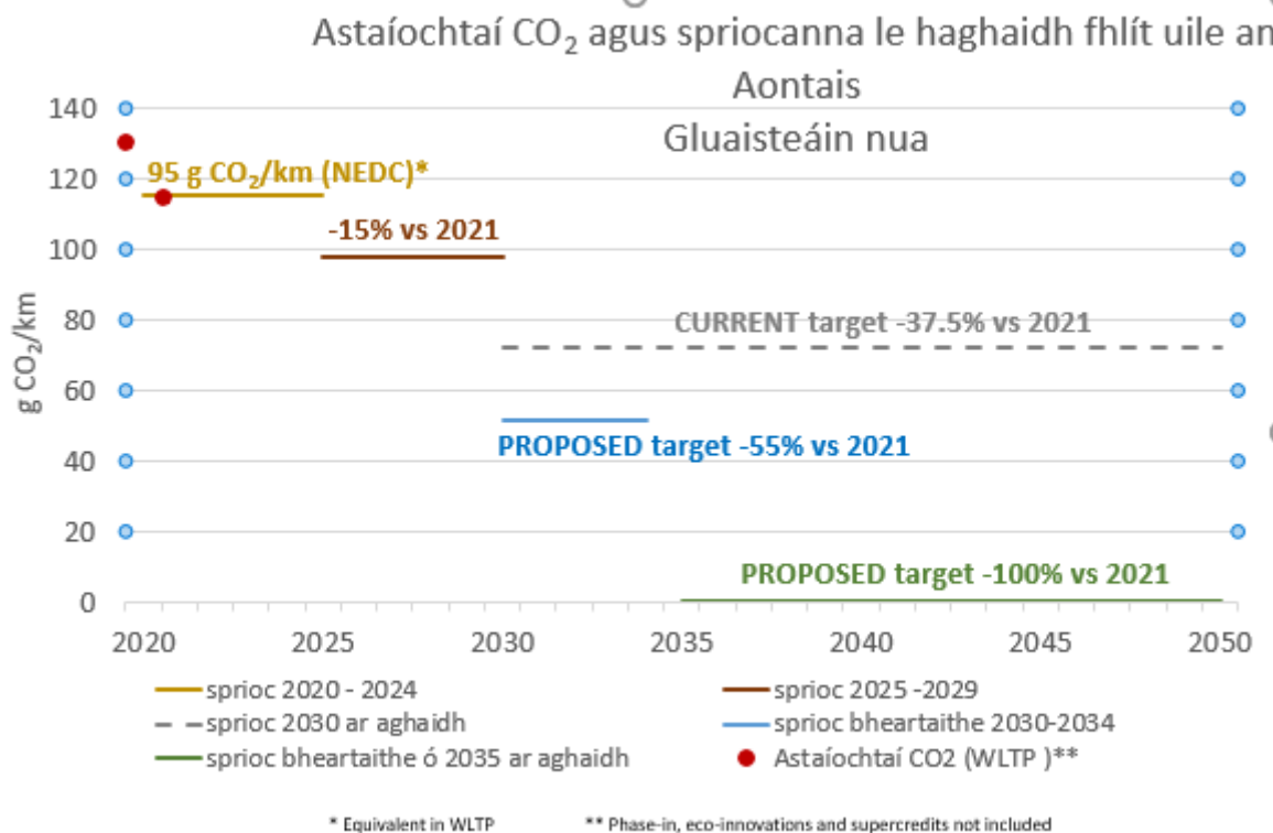
Fíor 9: Astaíochtaí CO 2 agus spriocanna le haghaidh fhlít uile an Aontais, gluasteáin agus veaineanna
