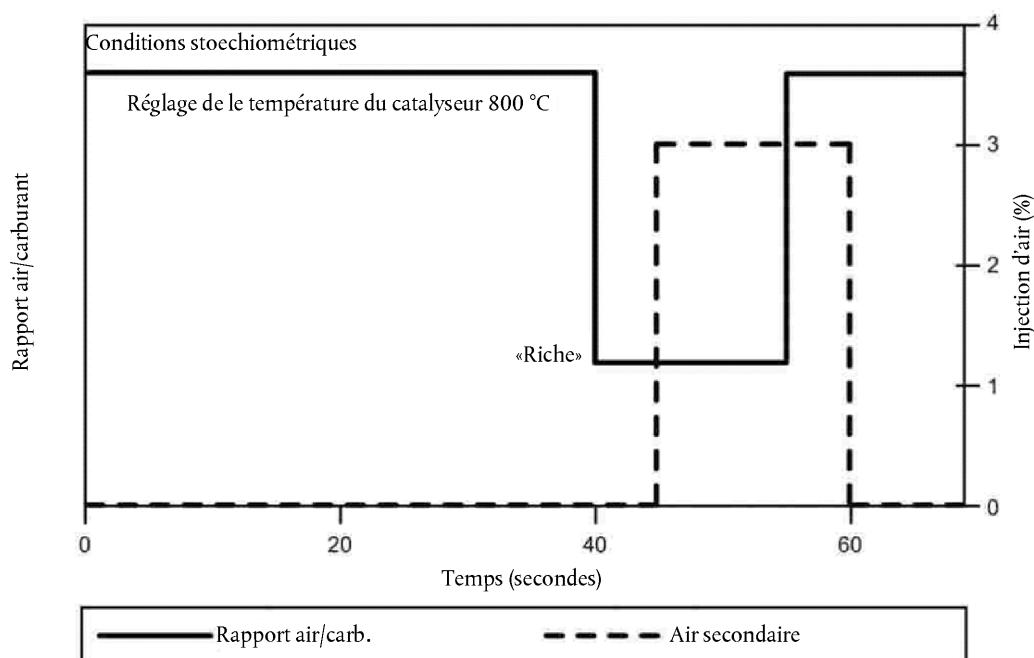
Cycle normalisé sur banc
