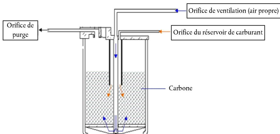
Schéma de circulation gazeuse et orifices de la cartouche de carbone
