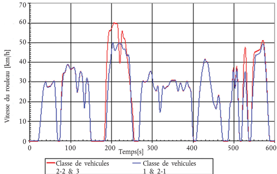
Première partie du cycle WMTC phase 2
