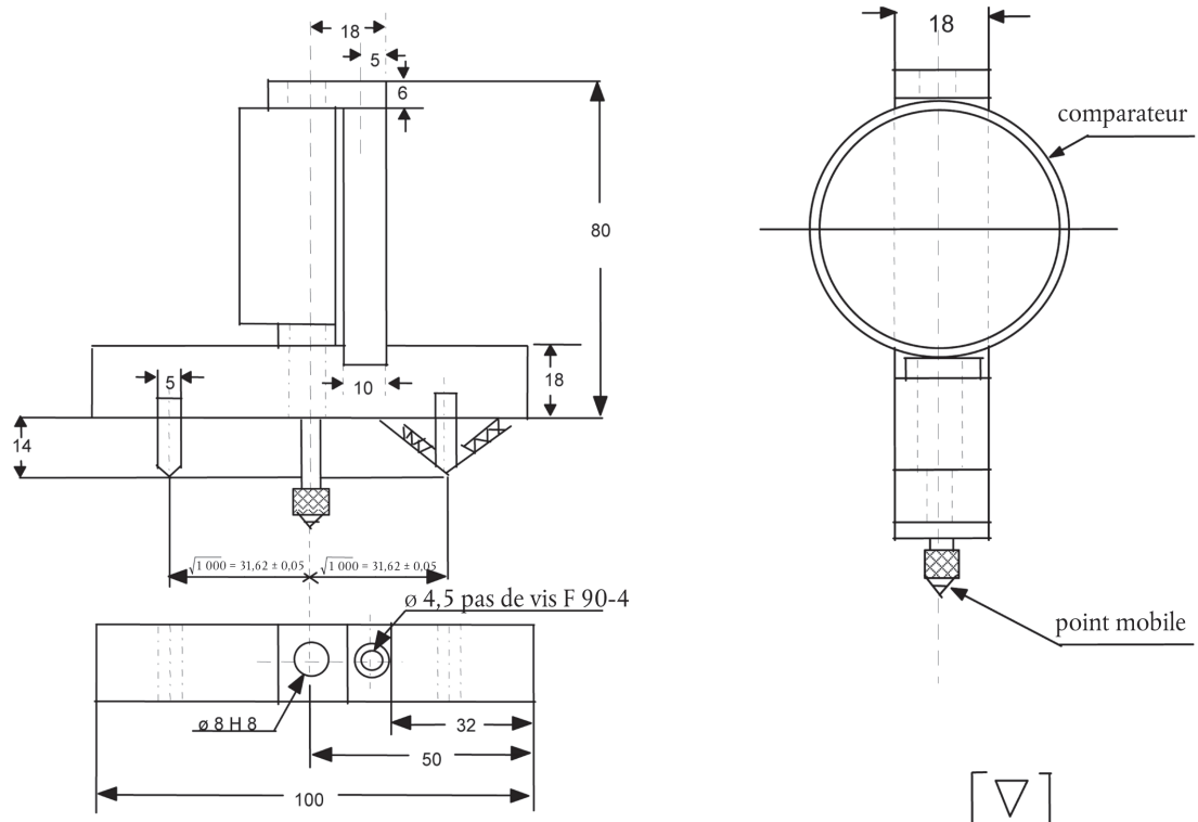
Figure 3 — Sphéromètre
