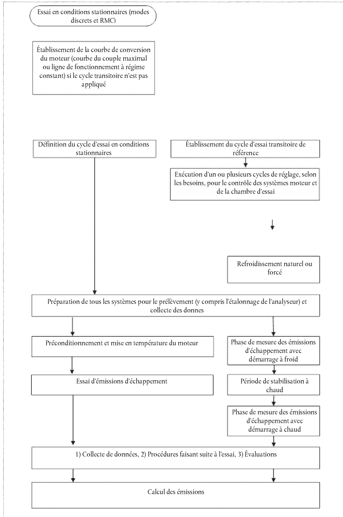
Figure 6.4 Séquence d'essai
