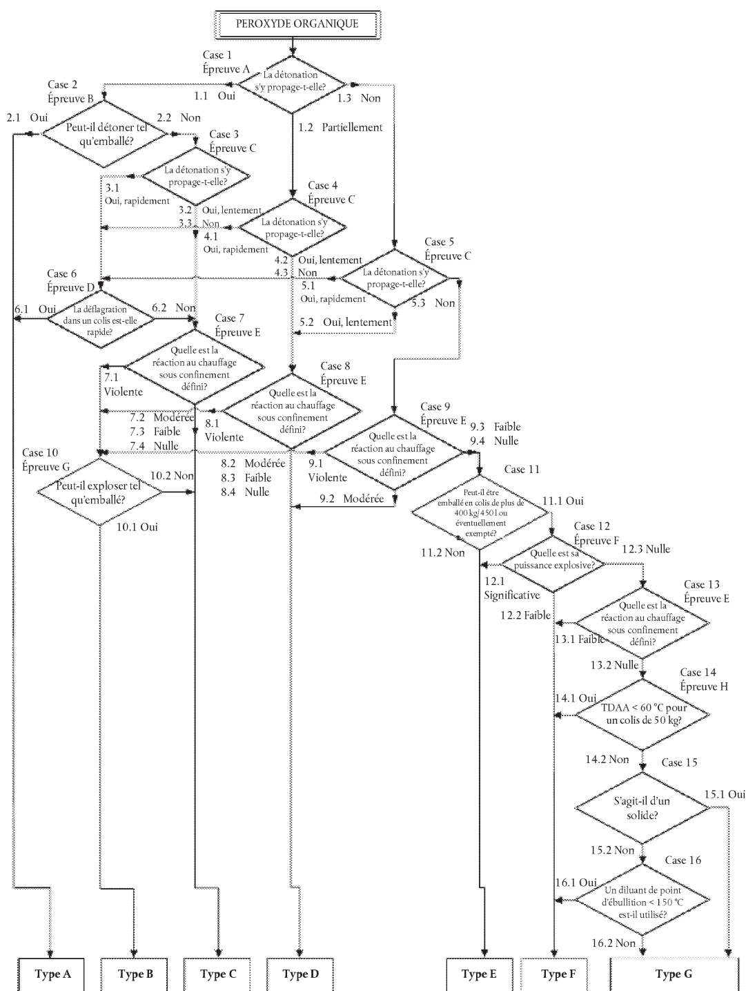
Figure 2.15.1 Peroxydes organiques
