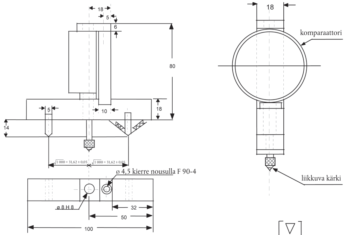
Kuvio 3: Pallon säteen mittauslaite
