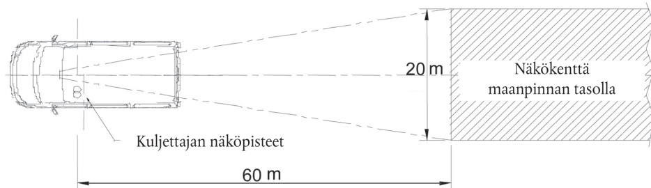
Kuvio 6: Luokan I peilin näkökenttä
