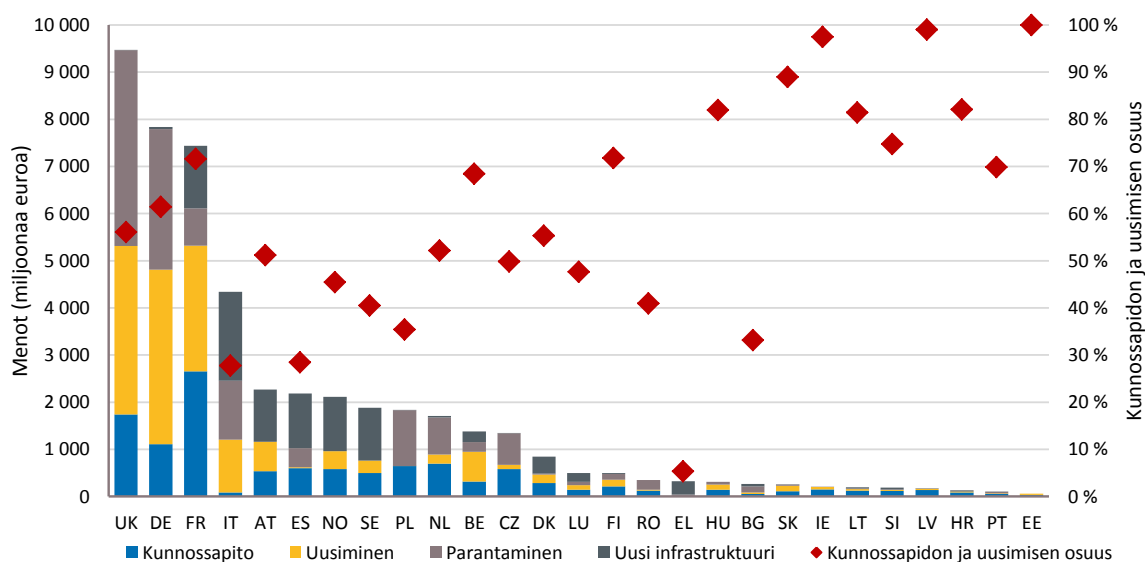
Kuva 11: Infrastruktuurimenot sekä kunnossapidon ja uudistamisen osuus maittain vuonna 2016
