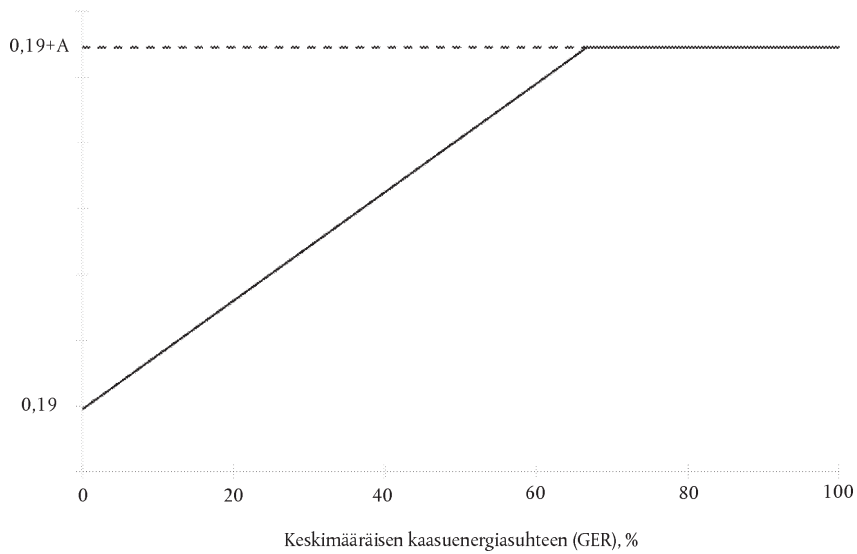
Kuva 1. Kaavio hiilivetyypäästörajasta keskimääräisen kaasuenergiasuhteen (GER) funktiona
