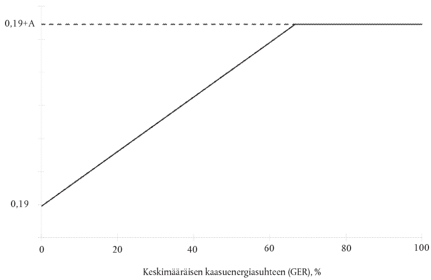
Kuva 1. Kaavio hiilivetyypäästörajan keskimääräisen kaasuenegiasuhteen (GER) funktiona
