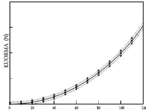
Kuva Ap3-1 alustadynamometrin absorboima teho
