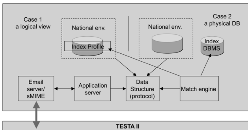
Joonis 2: Rakenduse topoloogia ülevaade
