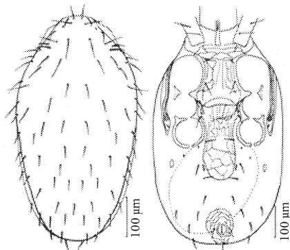
Hypoaspis aculeifer Hughesi järgi (Hughes, 1976)
