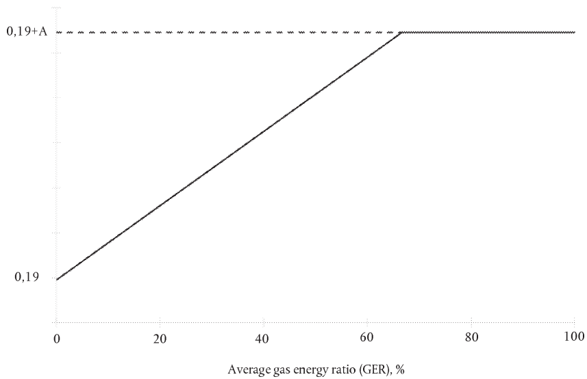
Joonis 1. Süsivesinike (HC) heite piinormi skeem GER-funktsioonina.
