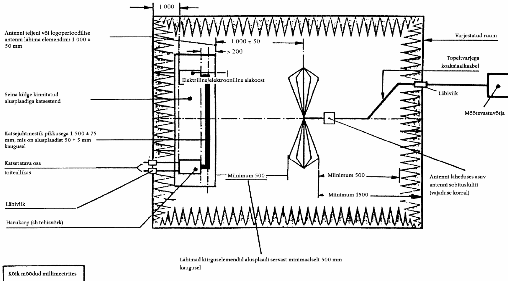
Elektrilise/elektroonilise alakoostu elektromagnetkiirguse katseskeem (ülevaade)
