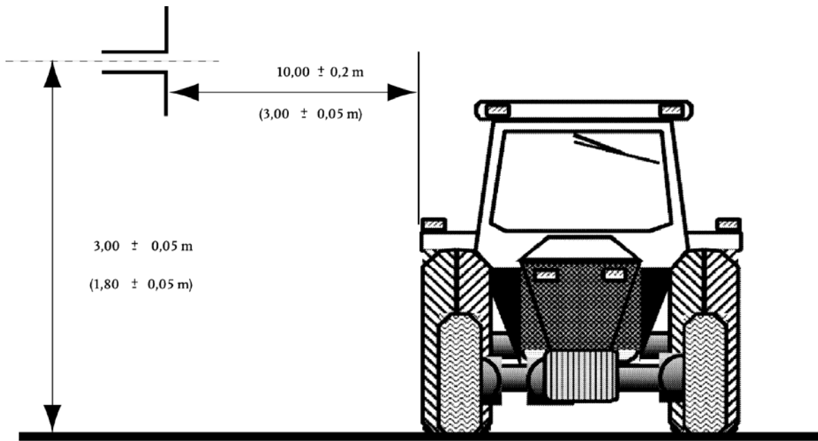
Joonis 2 ANTENNI ASEND TRAKTORI SUHTES
