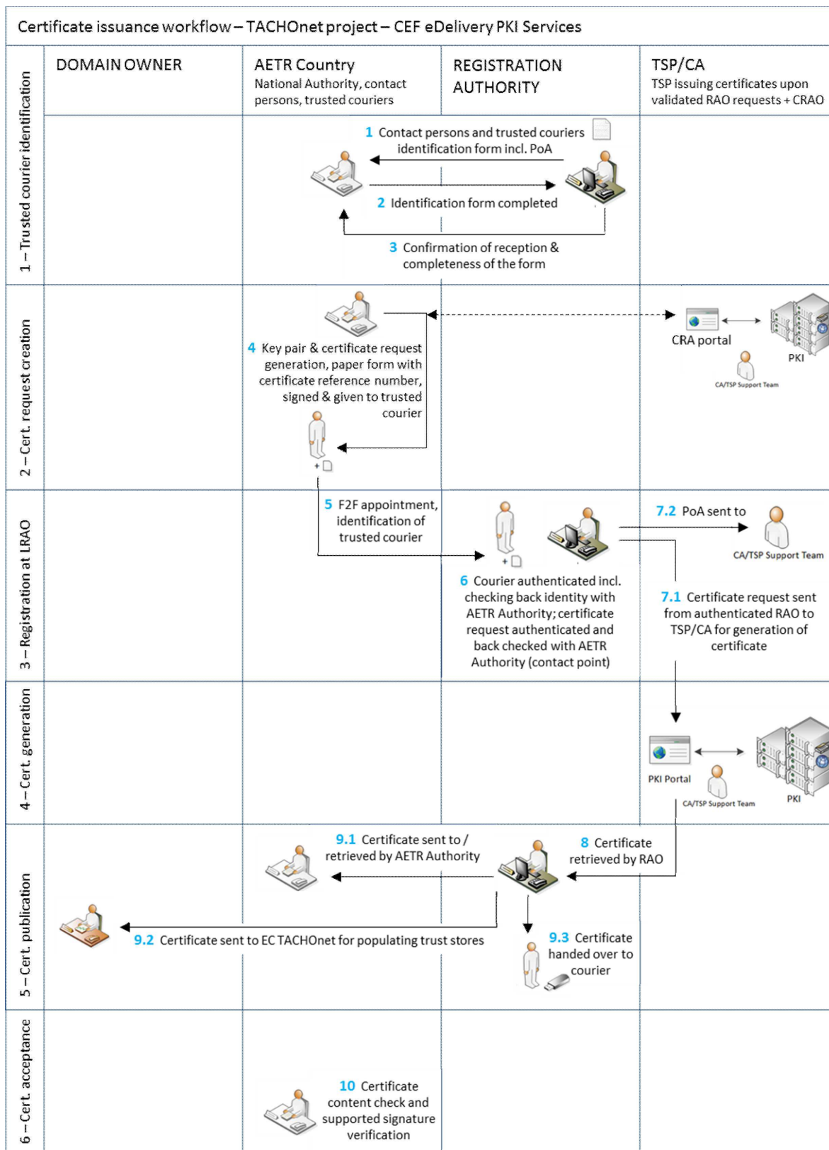
Joonis 1 – Sertifikaadi väljaandmise töövoog
