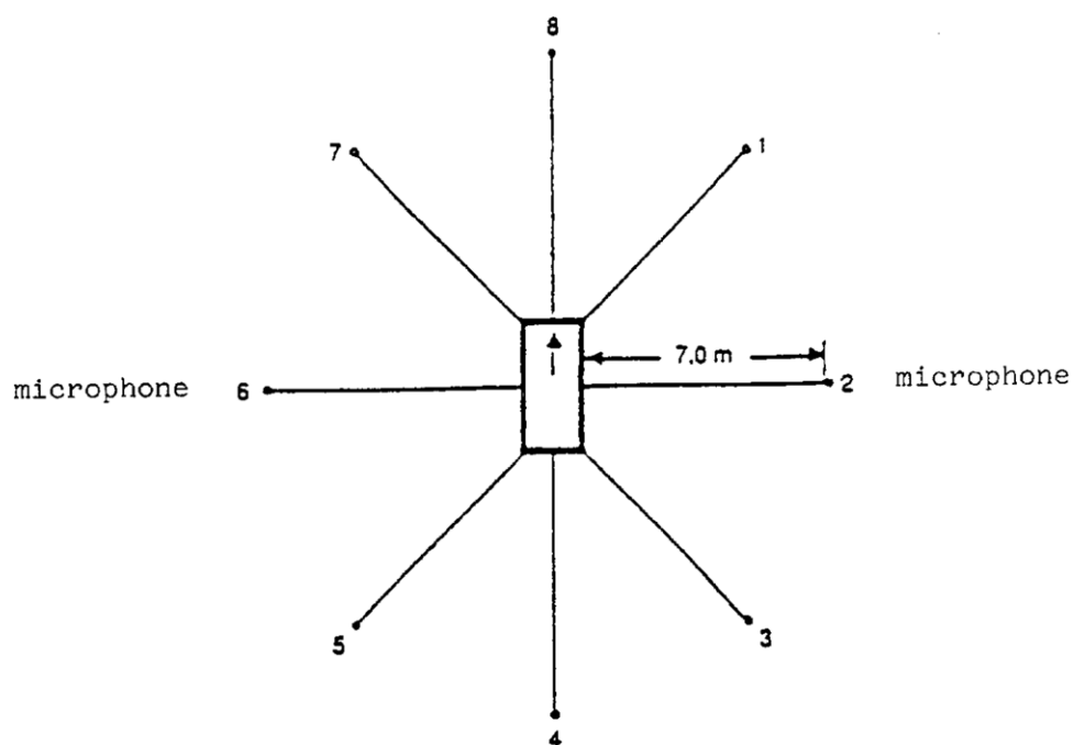
Joonis 1. Mikrofoni asendid suruõhumüra mõõtmisel
