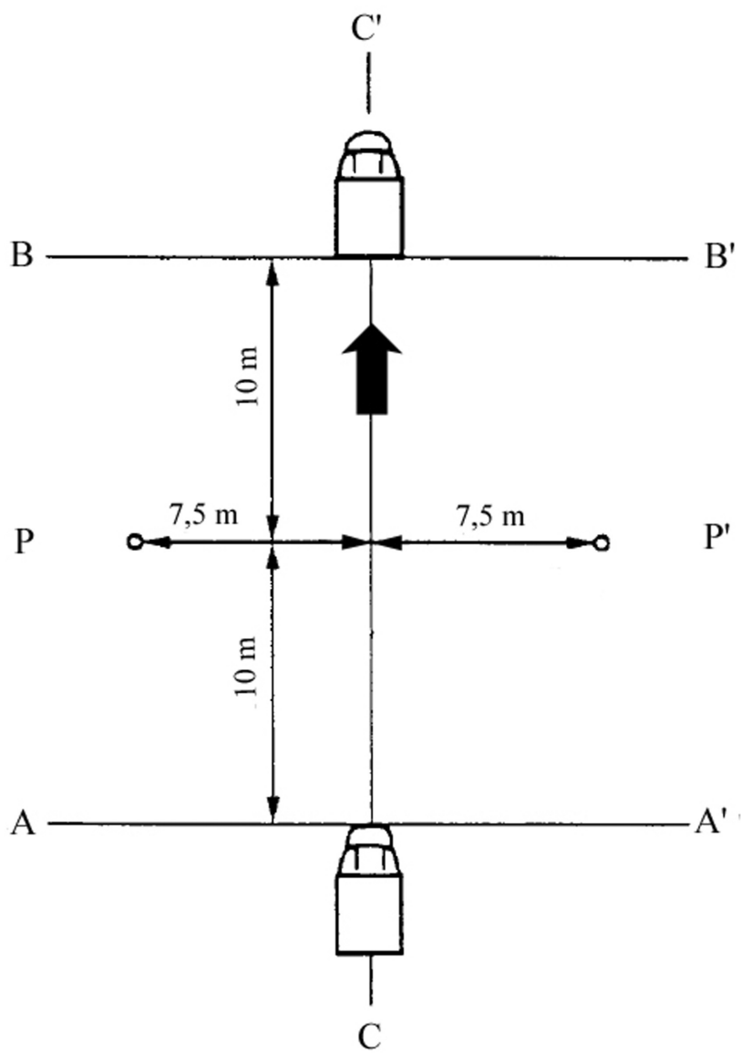
Joonis 1. Liikuvate sõidukite mõõtmisasendid
