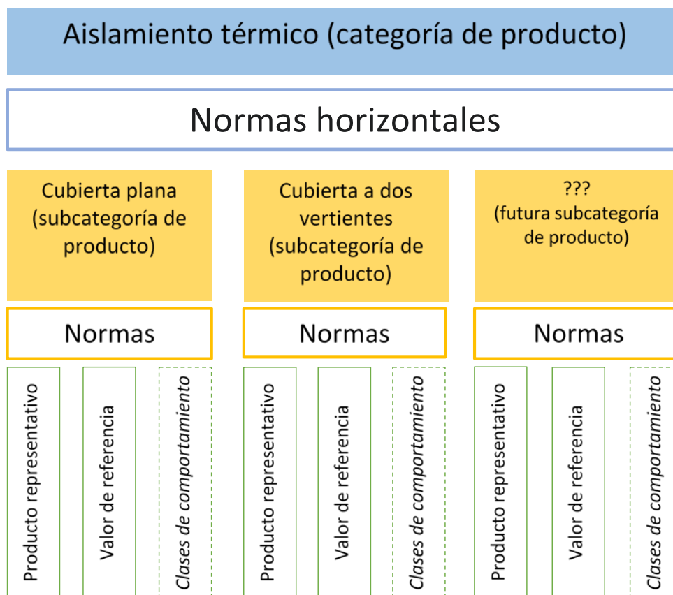
Gráfico L-3: Ejemplo de estructura de una RCHAP con normas horizontales específicas de la categoría de producto, diversas subcategorías de producto y normas verticales específicas de la subcategoría de producto.
