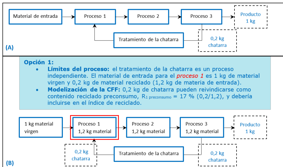
Gráfico 6: Opción de modelización cuando se alega que la chatarra preconsumo es contenido reciclado preconsumo
