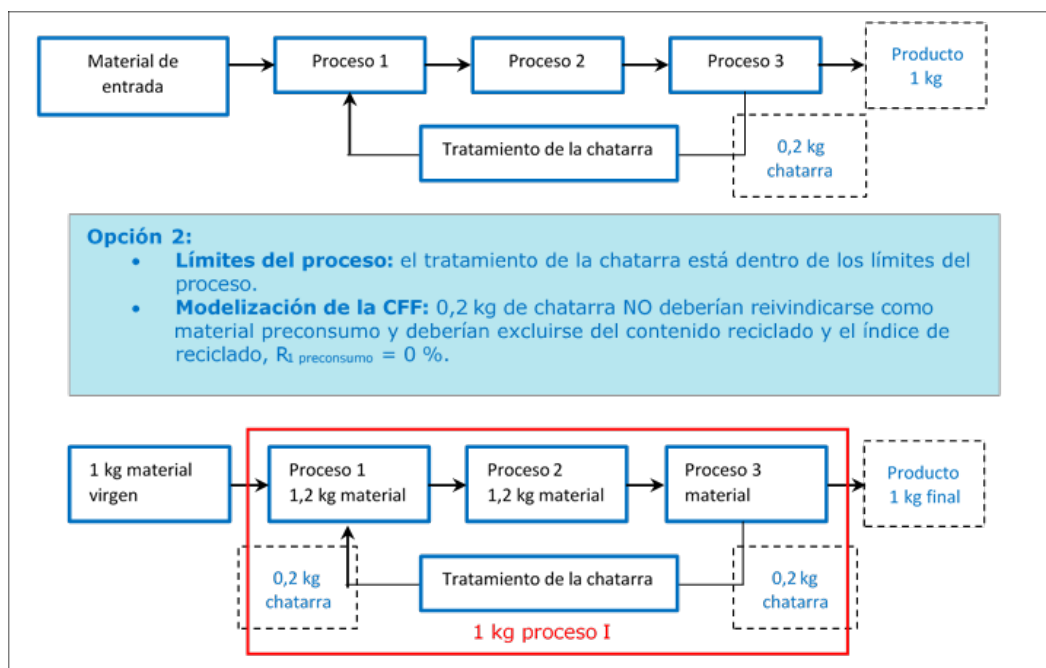
Gráfico 8: Opción de modelización cuando no se alega que la chatarra preconsumo es contenido reciclado preconsumo
