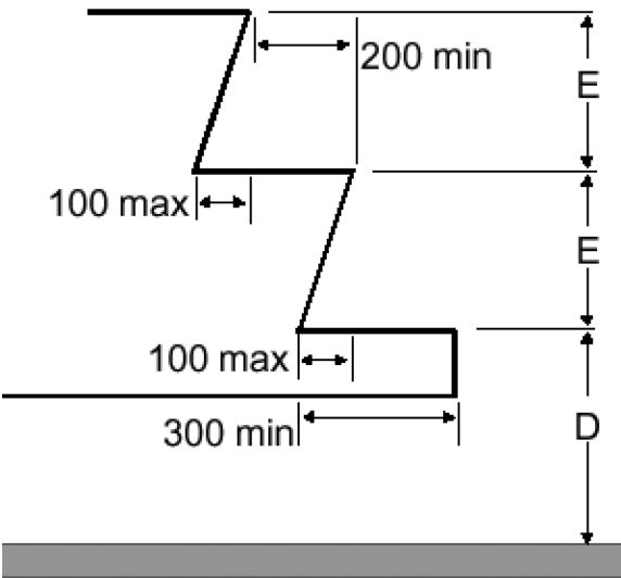
Figura 8 Escalones para viajeros (véase el anexo 3, punto 7.7.7)
