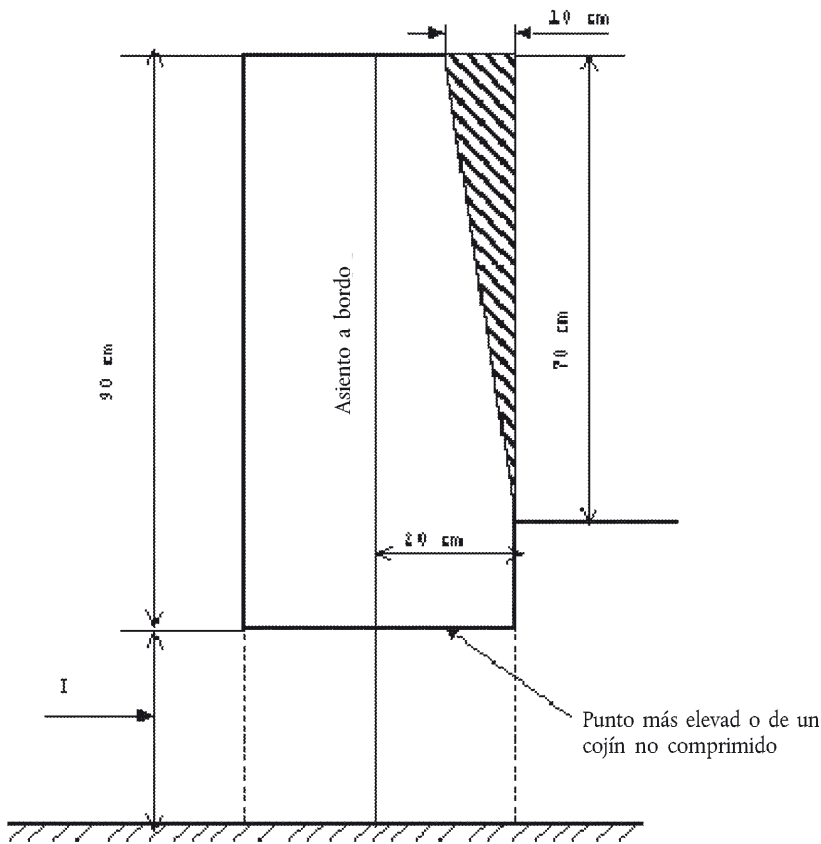
Figura 15 Intrusión permitida por encima del asiento (véase el anexo 3, punto 7.7.8.6.3.2)
