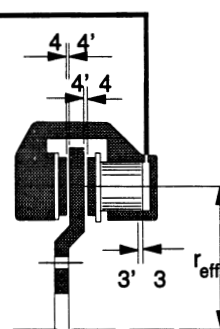
Freno de disco
