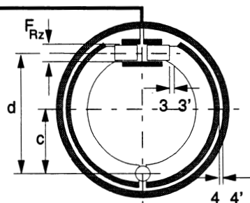
Freno de tambor
