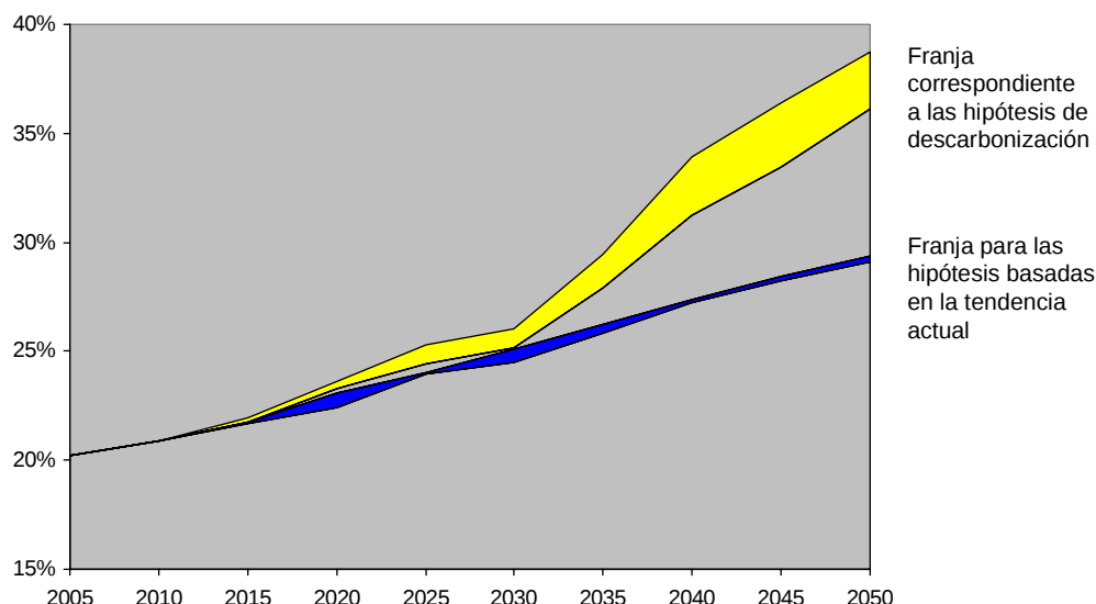
Gráfico 2: Cuota de electricidad en las hipótesis basadas en la tendencia actual y en las hipótesis de descarbonización (en % de la demanda final de energía)
