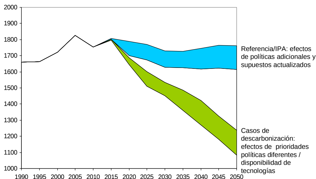
Gráfico 3: Consumo bruto de energía – Franja correspondiente a las hipótesis basadas en la tendencia actual (REF/IPA) y a las hipótesis de descarbonización (en Mtep)
