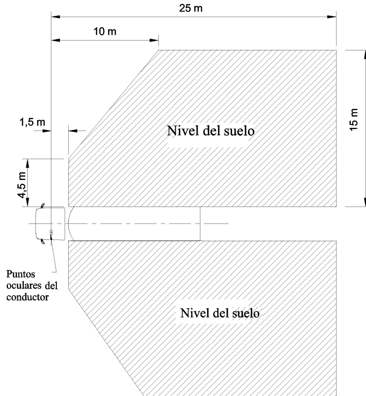
Figura 9: Campo de visión de un retrovisor exterior gran angular de la clase IV
