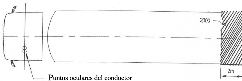
Figura 12: Campo de visión de los dispositivos posteriores de visión indirecta
