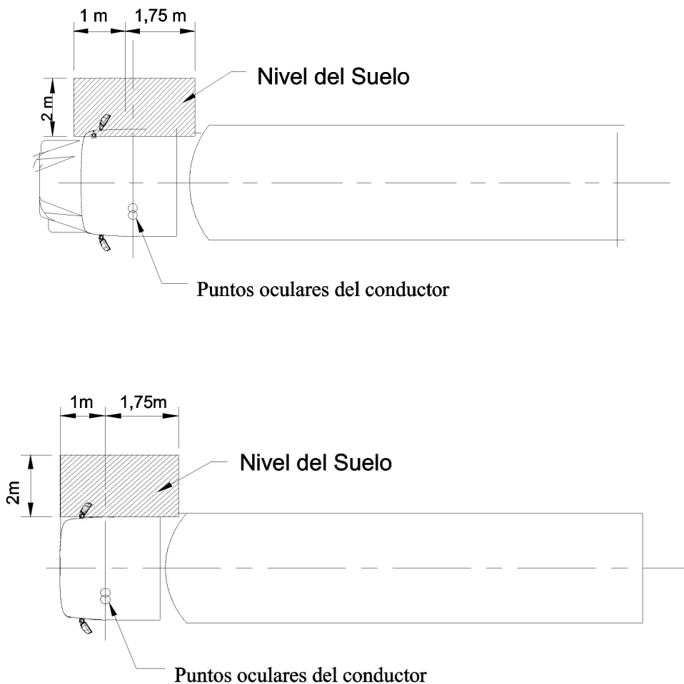
Figuras 10a y 10b: Campo de visión de un retrovisor de proximidad de la clase V
