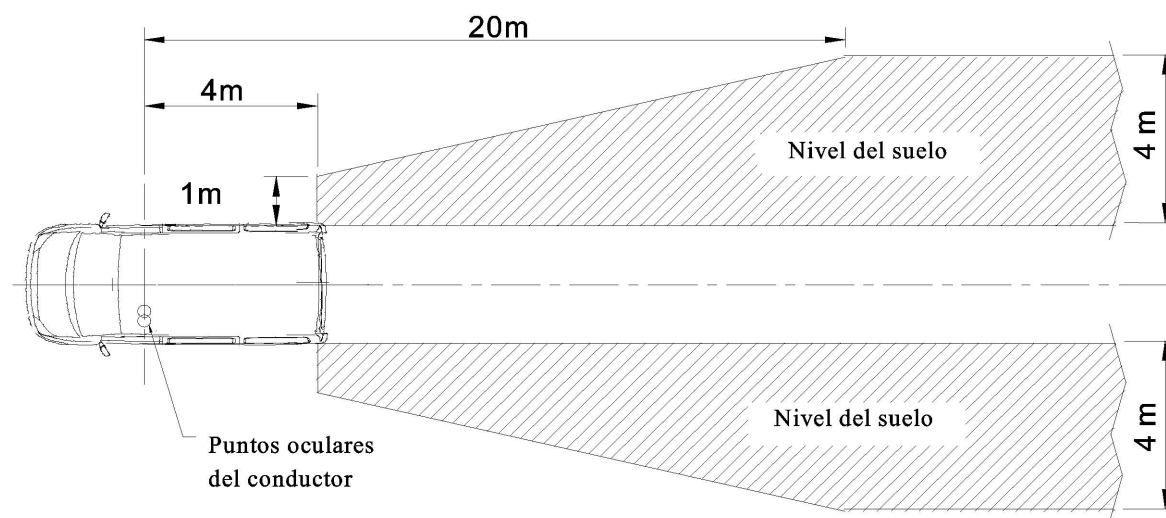
Figura 8: Campo de visión de un retrovisor de la clase III
