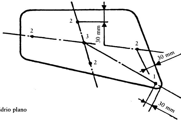
2 a) Placa de vidrio plano
