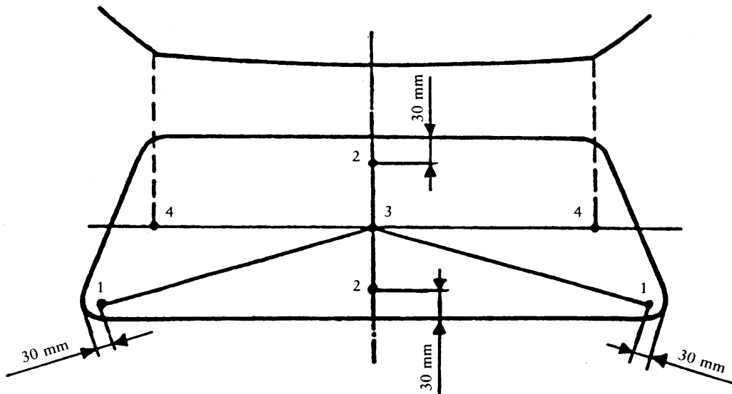
2 c) Placa de vidrio curvado
