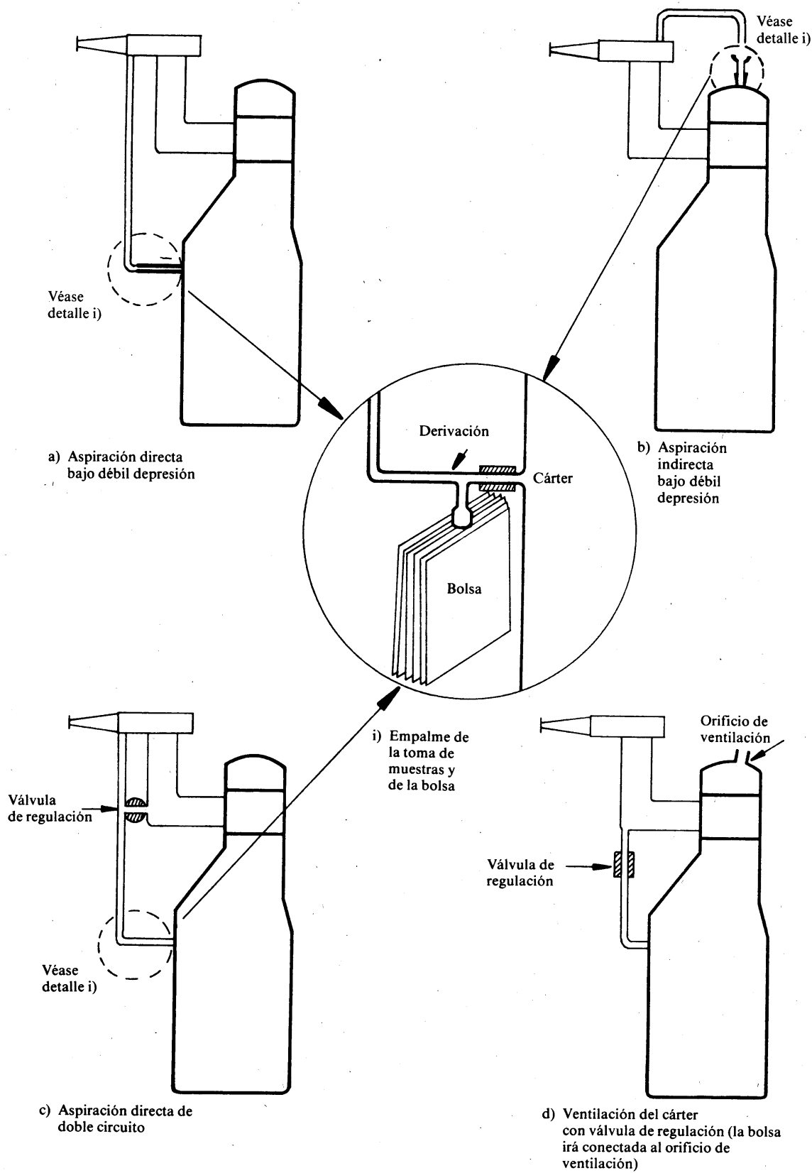
Figura V/5 Prueba del tipo III
