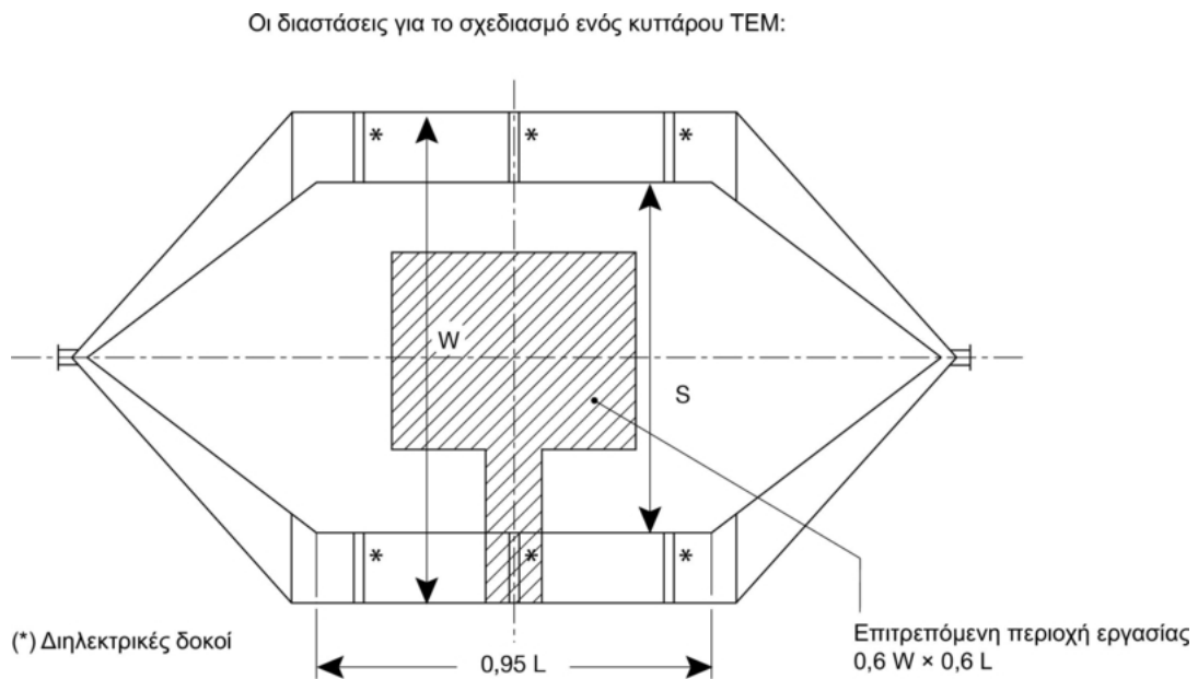
Εικόνα 2 Διαστάσεις κυττάρου TEM
