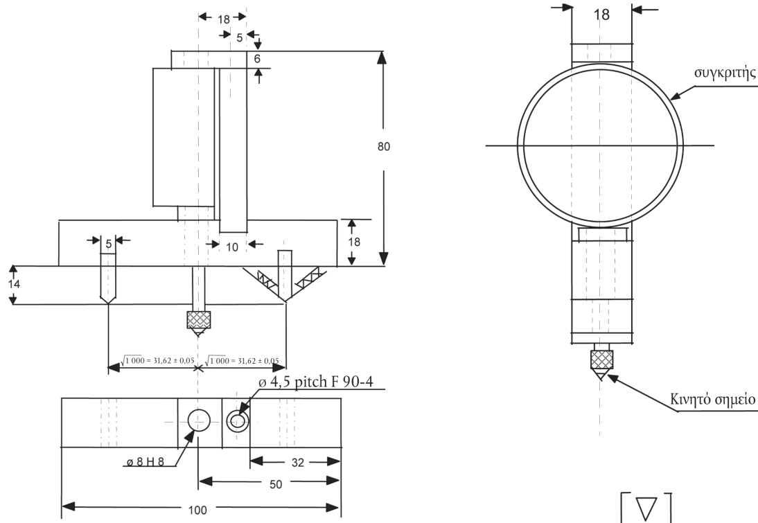
Σχήμα 3: σφαιρόμετρο
