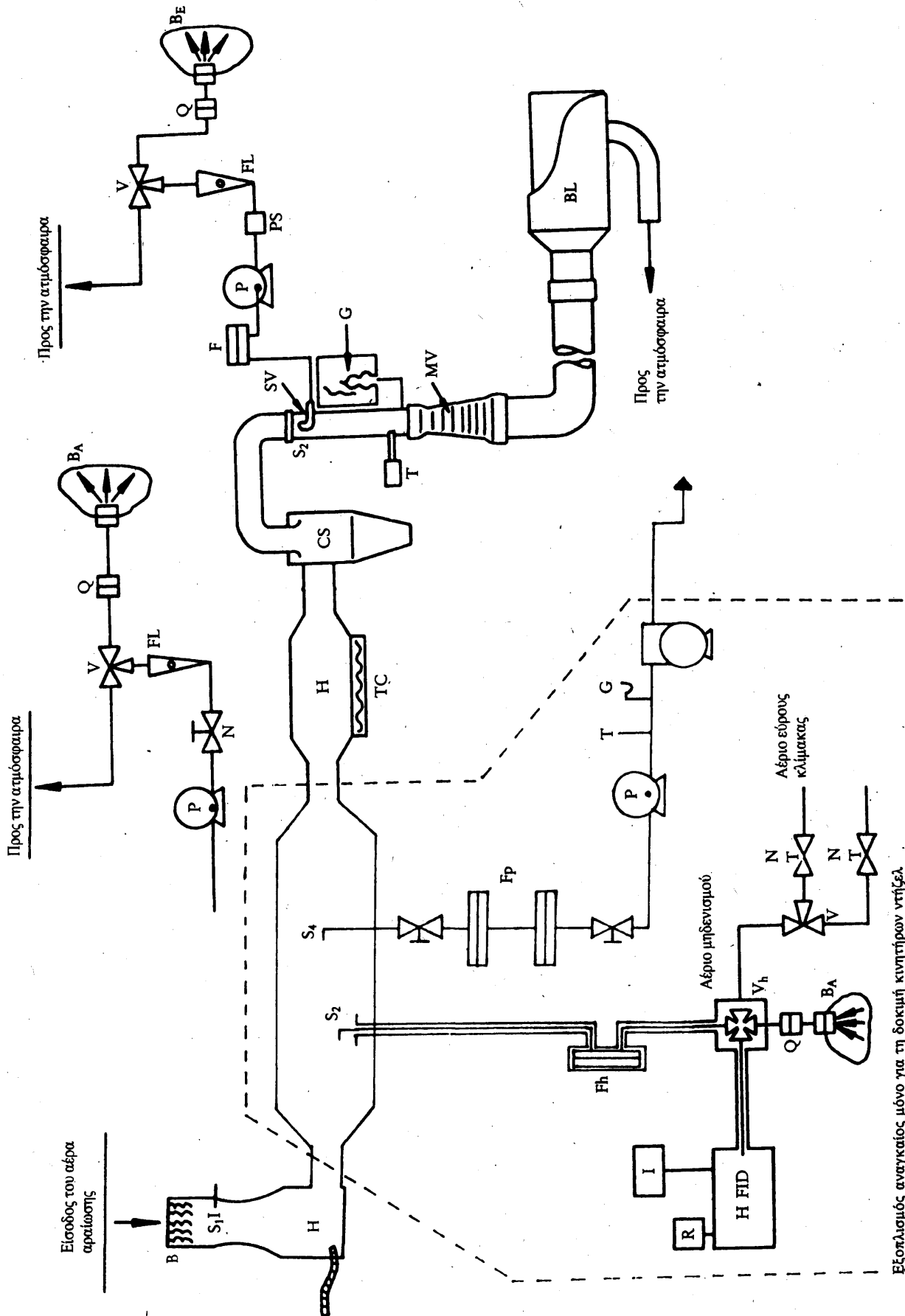
Σχήμα III/5.3.2 Διάγραμμα συστήματος δειγματοληψίας υπό σταθερό όγκο με σωλήνα Venturi κρίσιμης ροής (σύστημα CFV-CVS)
