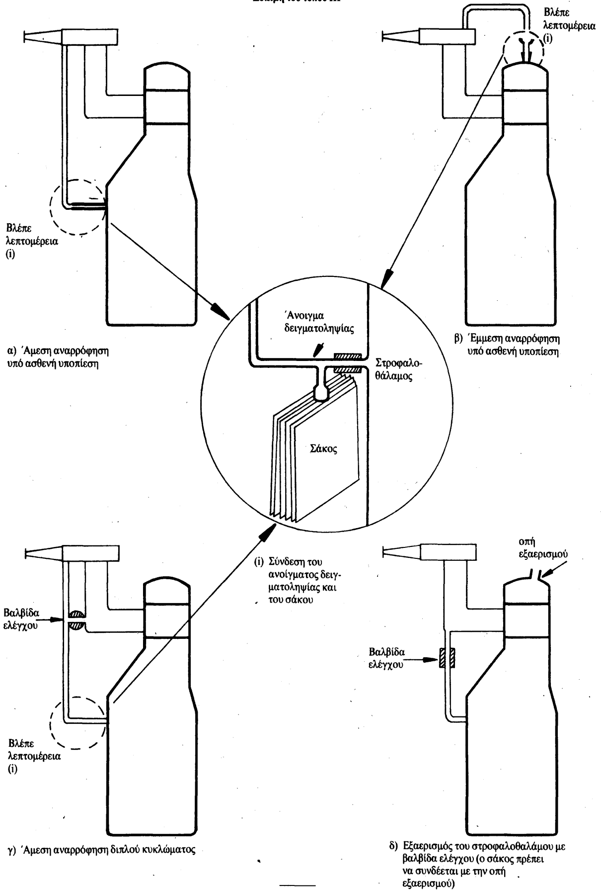
Σχήμα V/5 Δοκιμή του τύπου III
