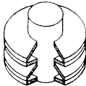
Ελατήριο επάλληλων δίσκων (τομή)
