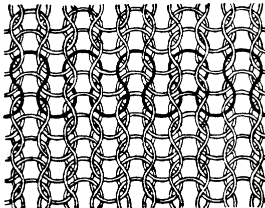
Σχήμα 9 Interlock
