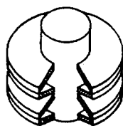
Ελατήριο επάλληλων δίσκων (τομή)
