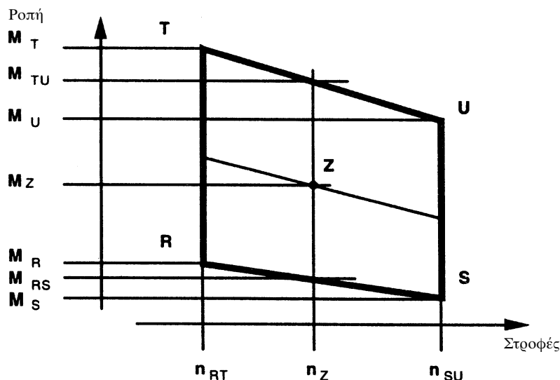
Παρεμβολή του σημείου ελέγχου των NO x
