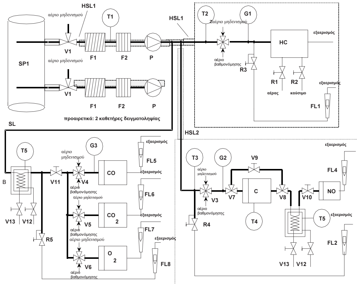
Διάγραμμα ροής συστήματος ανάλυσης καυσαερίων CO, NOx και HC
