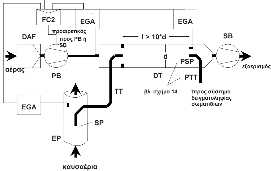
Σχήμα 6 Σύστημα αραιώσεως μερικής ροής με CO 2 και NO x και μέτρηση συγκεντρώσεων με κλασματική δειγματοληψία
