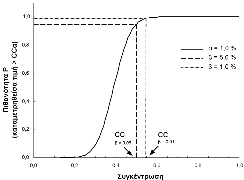
Σχήμα 1 Καμπύλη ισχύος
