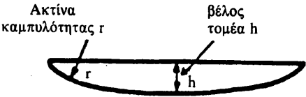
Περιγραφή των παραμέτρων r και h του αλεξήνεμου
