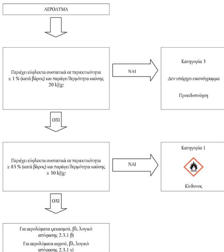
Διάγραμμα 2.3.1 α) Για τα αερολύματα
