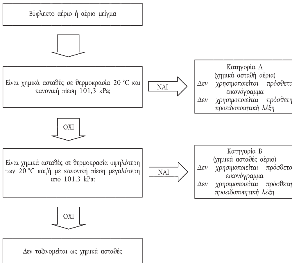
Διάγραμμα 2.2.2 Χημικά ασταθή αέρια
