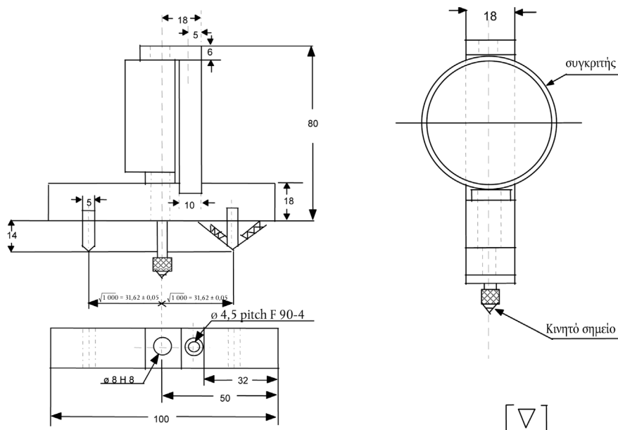
Σχήμα 3: σφαιρόμετρο
