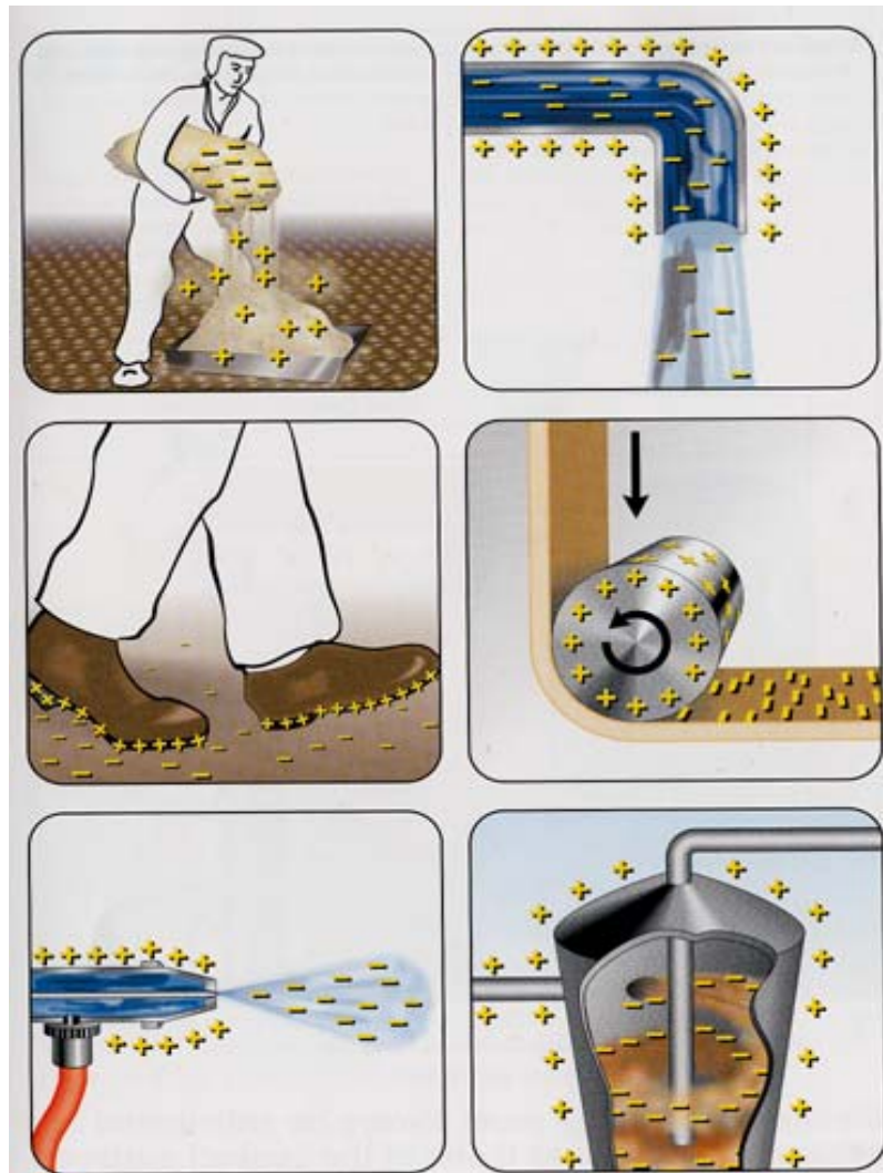
Abb. 3.6: Beispiele für Ladungstrennungen, die eine elektrostatische Aufladung bewirken können 4 .
