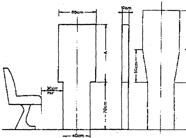
Abbildung 1 Zugang zu den Betriebstüren (siehe 7.7.1)
